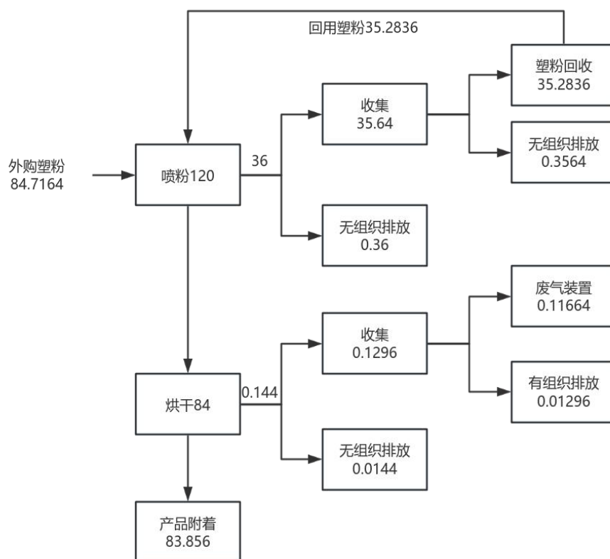
图 2-2 粉末涂料平衡图 (t/a)
