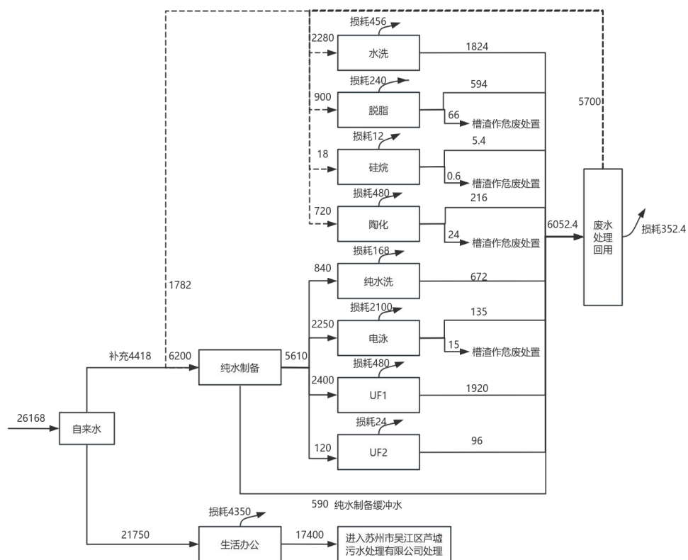
图 2-4 全厂水平衡图 (t/a)
