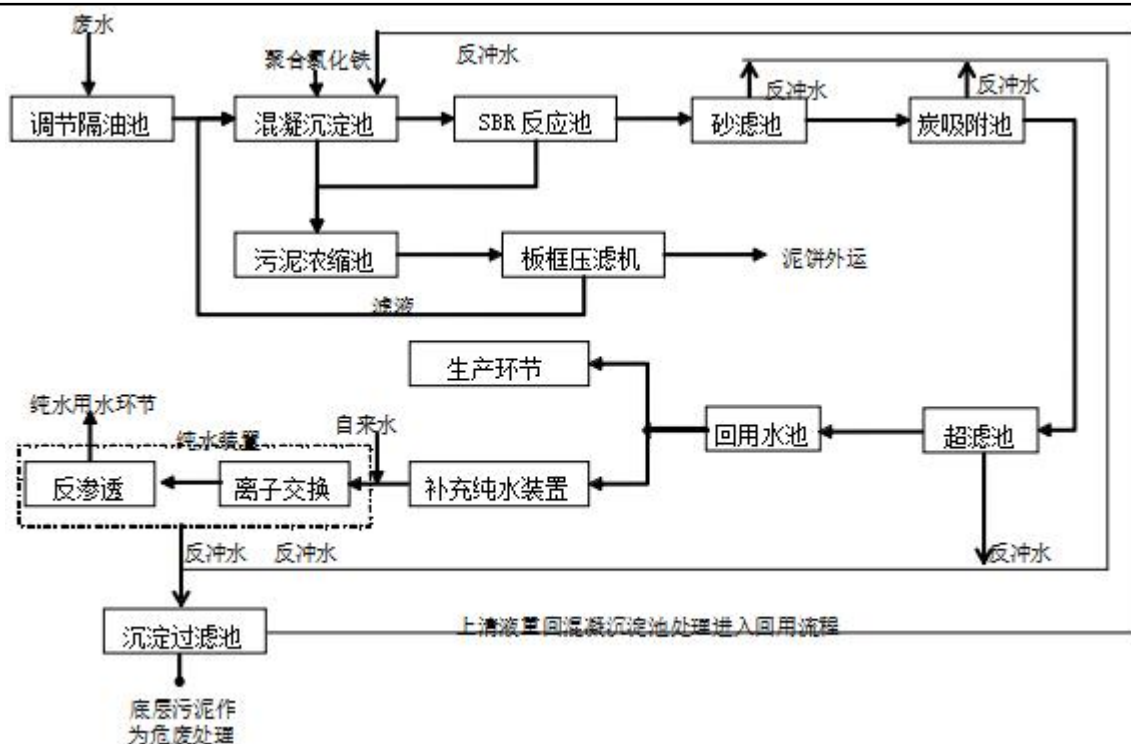
图 4-3 污水处理站处理工艺流程图
