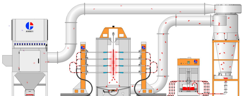
图 4-2 塑粉回收设备示意图
