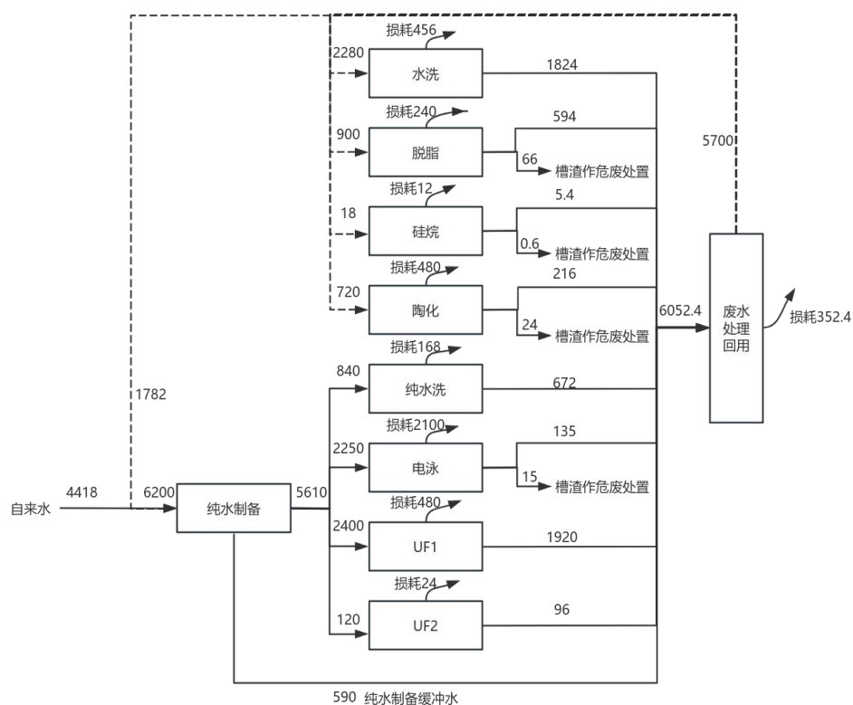
图 2-3 本项目水平衡图 (t/a)
