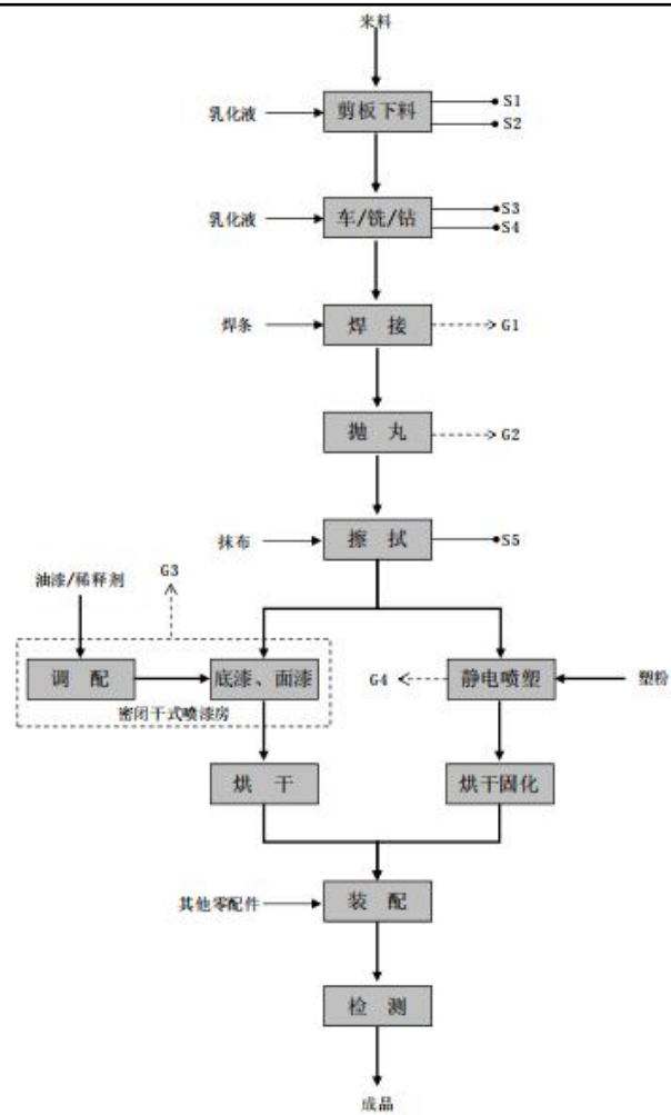
图 2-6 现有电梯、自动扶梯、人行道生产工艺流程
