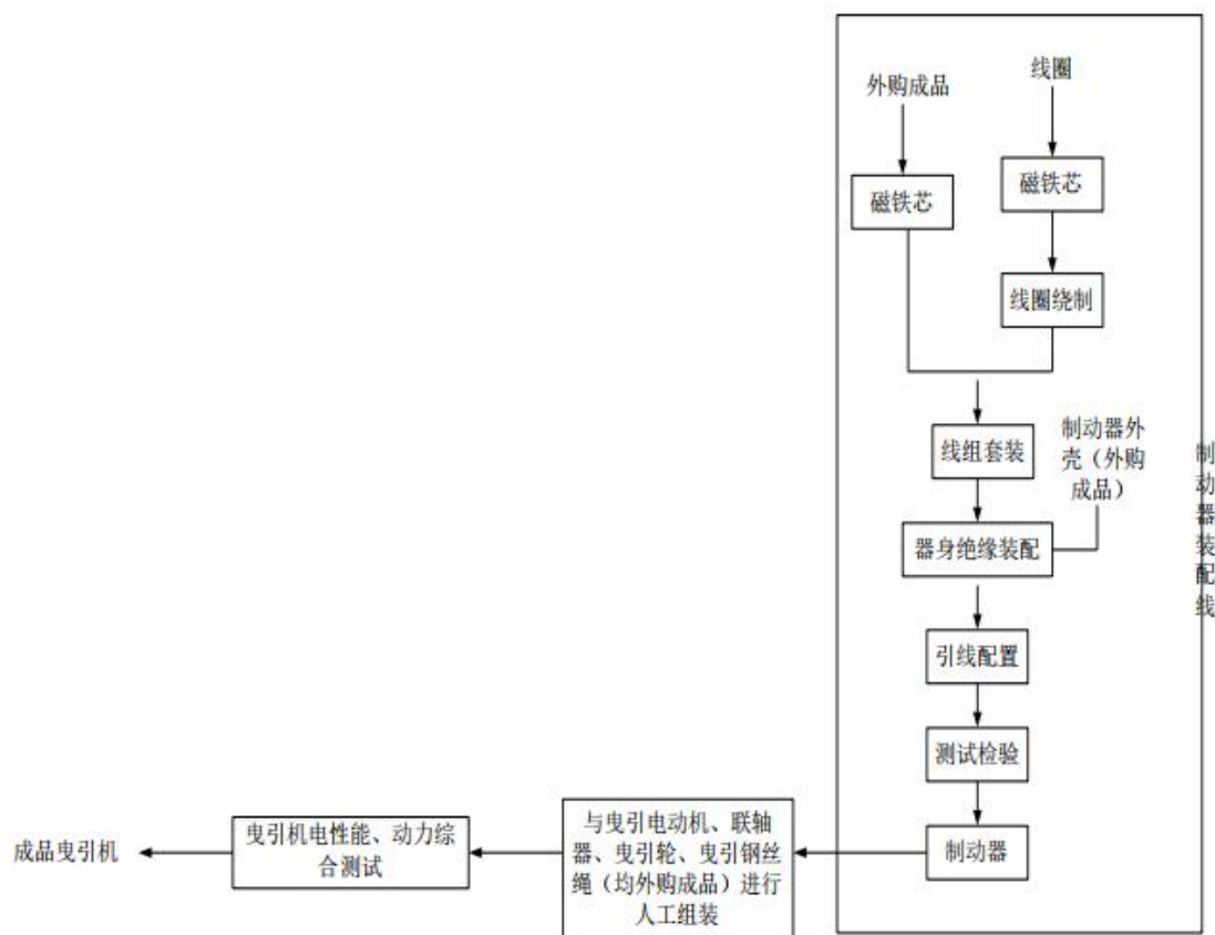
图 2-8 现有电梯曳引机生产工艺流程
