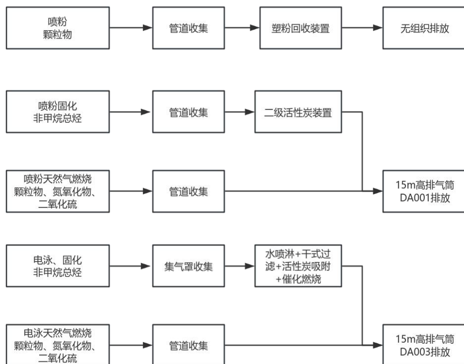
图 4-1 废气收集及处置系统示意图
