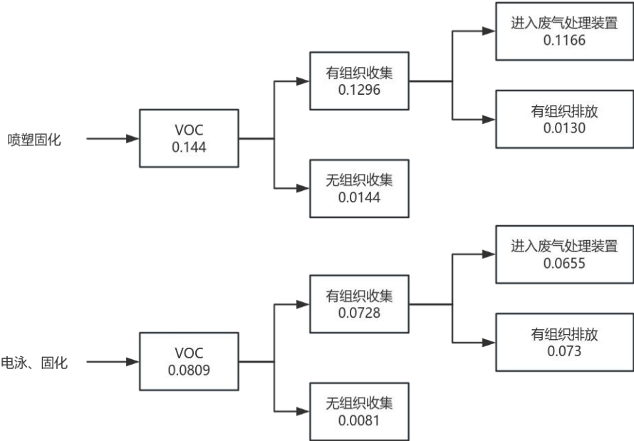
图 2-1 VOC 平衡图（t/a）
