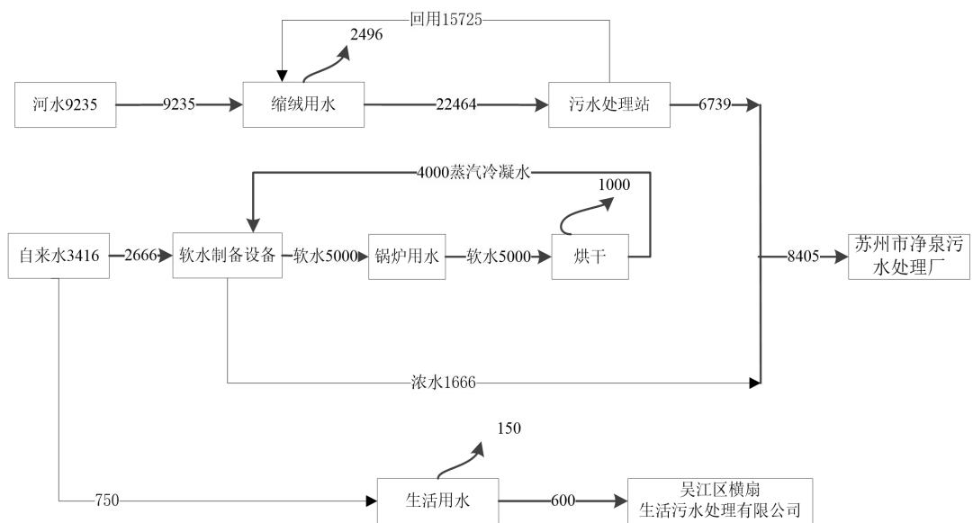
图 2-2 技改后水平衡图 (t/a)
