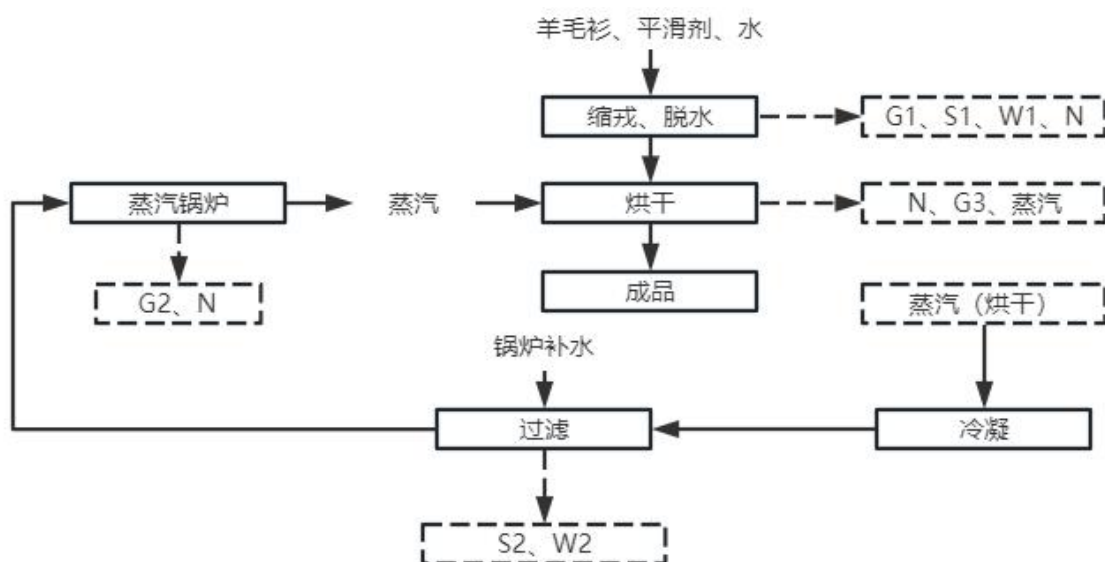
图 2-3 本项目生产工艺流程图
