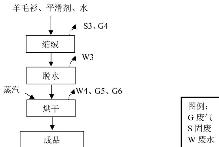
图 2-4 原有项目生产工艺流程图
