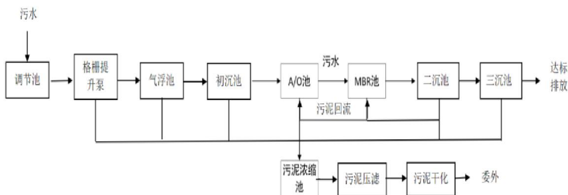
图4-3 苏州市净泉污水处理厂废水处理工艺流程图
