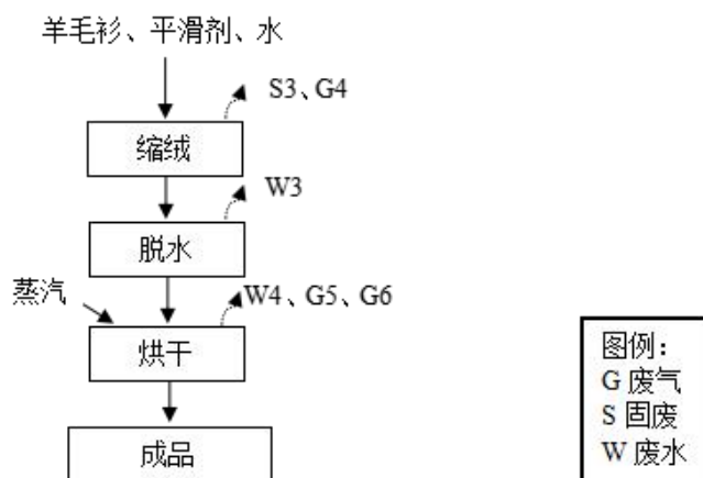
图 2-4 原有项目生产工艺流程图
