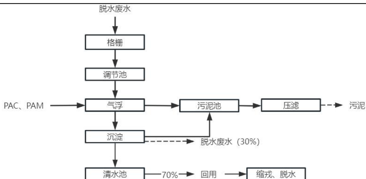
图 4-1 废水处理系统处理流程图
