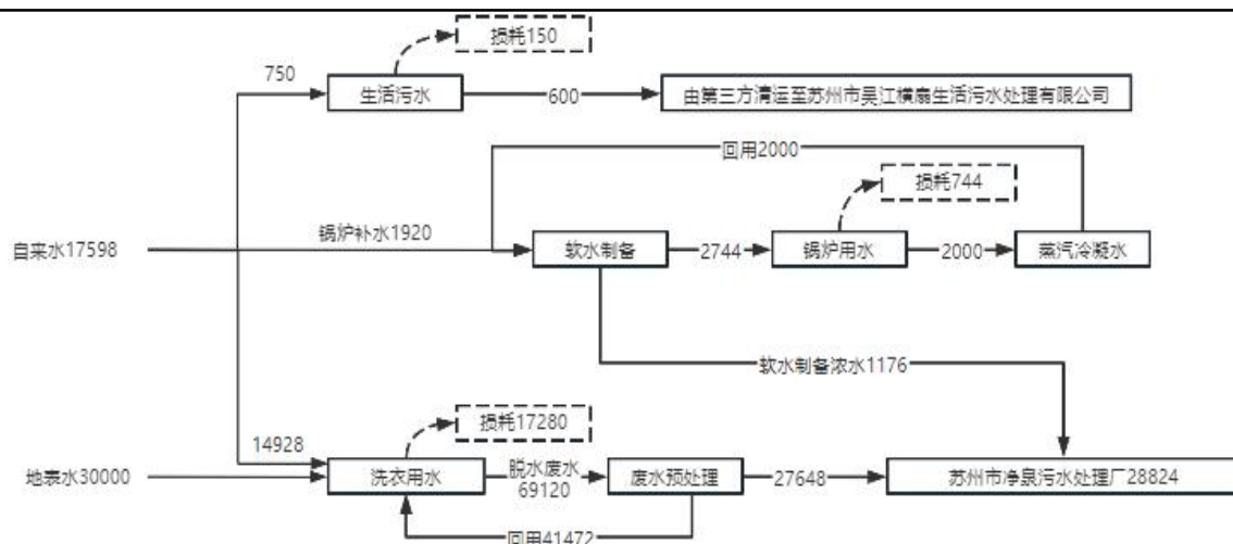
图2-1 技改前原有项目水平衡图 (t/a)
