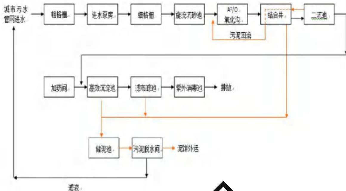
图 4-2 苏州市吴江横扇生活污水处理有限公司污水处理工艺流程图
