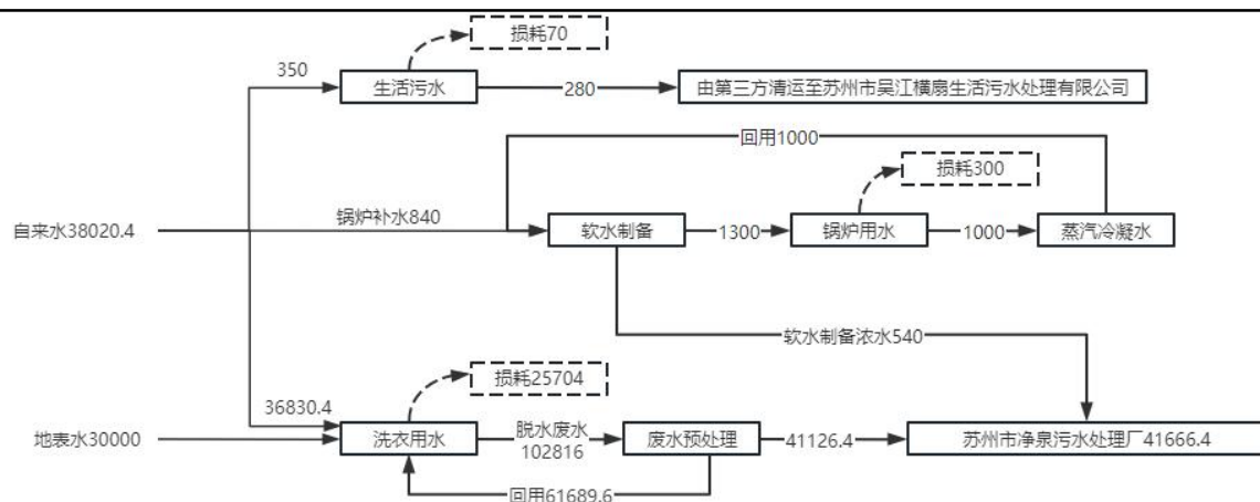
图2-1 技改前原有项目水平衡图 (t/a)
