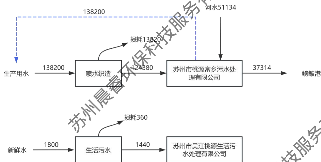
图 2-1 改建后全厂水平衡图 (t/a)
