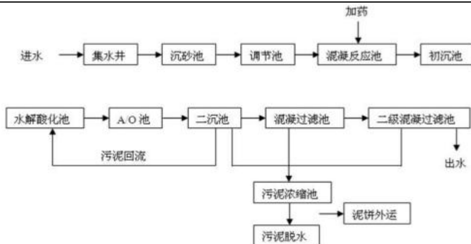
图 4-2 污水处理厂处理工艺图
