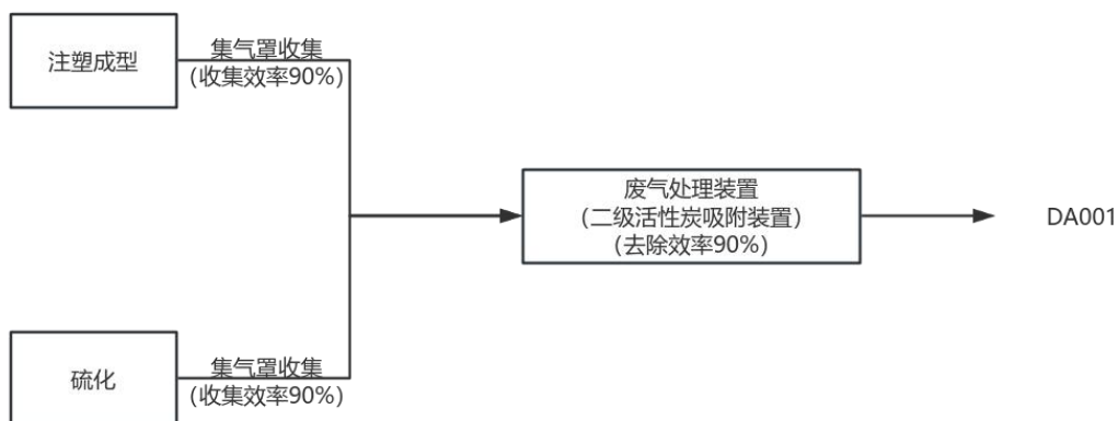
图 4-1 本项目废气收集及处理方式图
