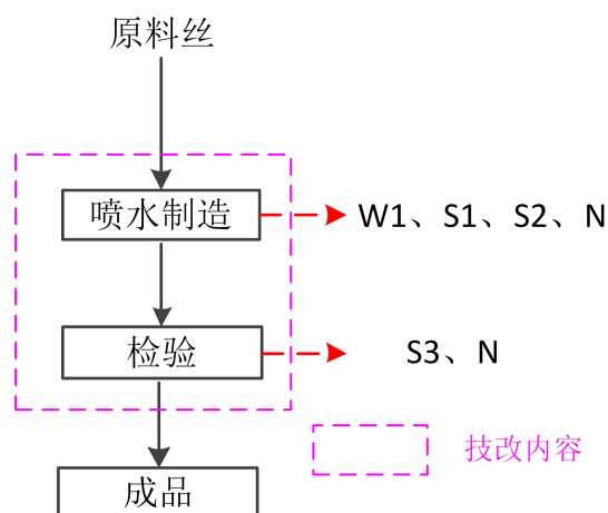
图 2-4 生产工艺流程及产污环节示意图
