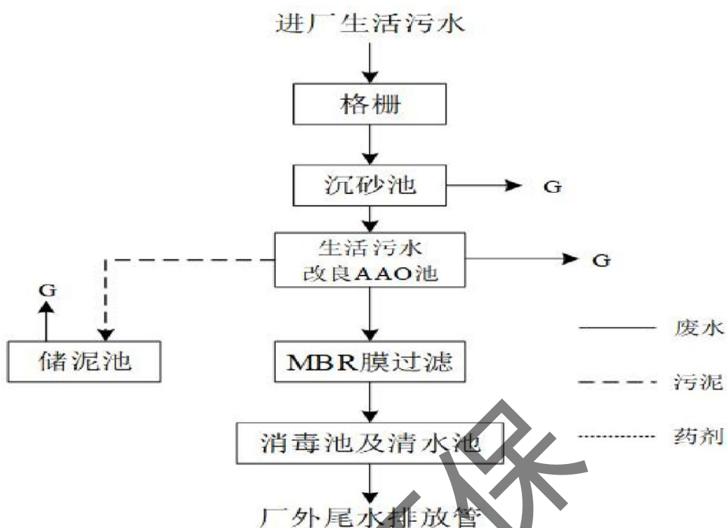
图 4-1 吴江市盛泽水处理发展有限公司（南部工业区综合污水处理厂）处理工艺流程
