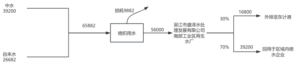
图 2-3 技改前吴江市盛誉喷织厂水平衡图 (单位 t/a)
