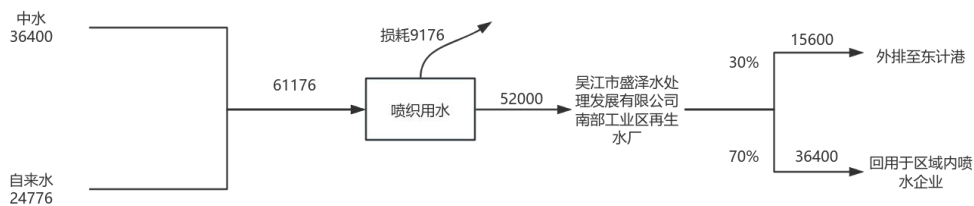
图 2-2 技改前吴江耀程纺织有限公司水平衡图 (单位 t/a)
