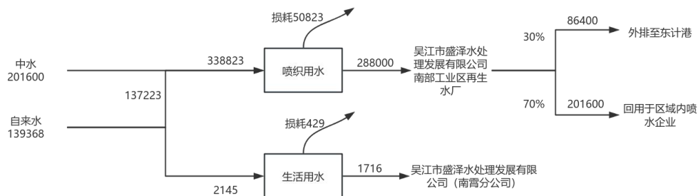
图 2-1 技改前吴江市永佳织造厂水平衡图 (单位 t/a)
