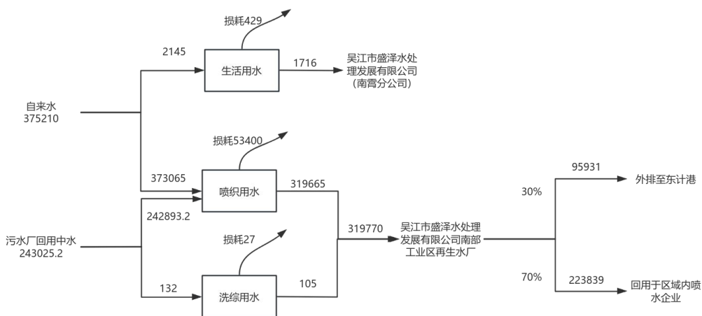
图 2-4 技改后水平衡图 (单位 t/a)
