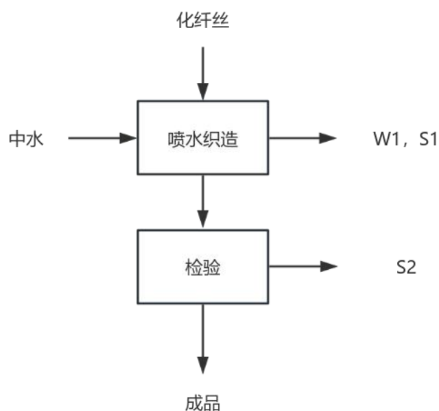
图 2-5 现有项目生产及产污环节示意图 W-废水 S-固废
