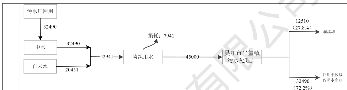
图2-5技改前吴江市意成织造有限公司水平衡图 t/a
