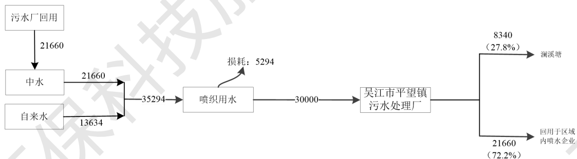
图2-2 技改前苏州丽龙芳纺织有限公司水平衡图 t/a
