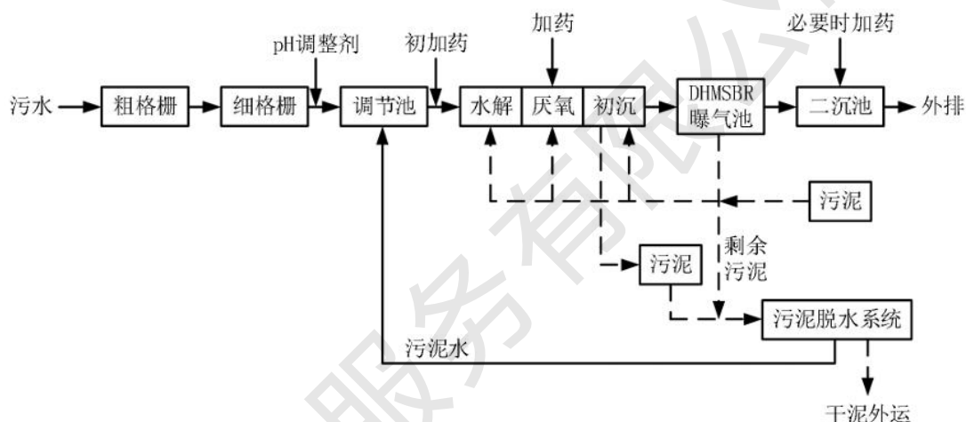
图 4-2 苏州市吴江平望生活污水处理有限公司工艺图
