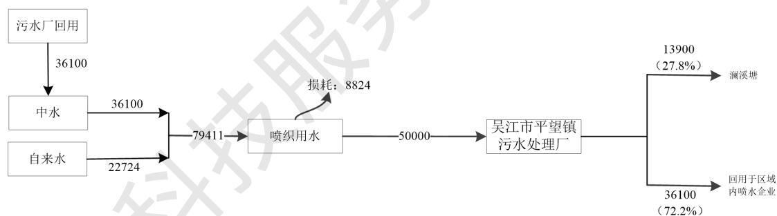
图2-6技改前苏州新方福纺织有限公司水平衡图 t/a
