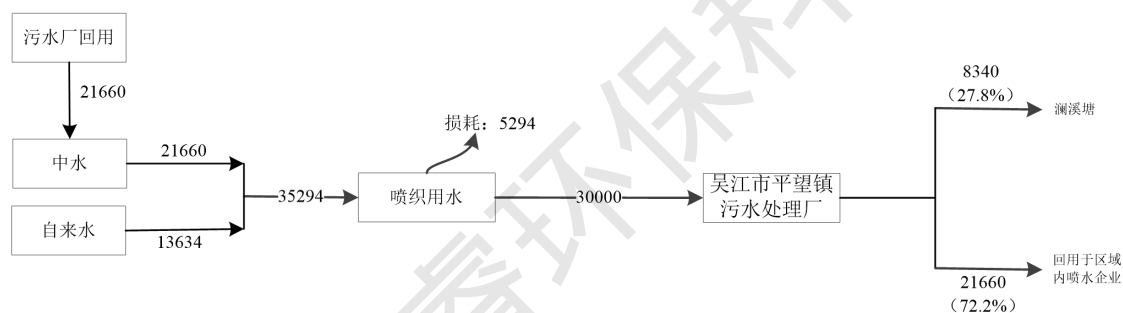
图2-8技改前苏州市诗妍琦纺织有限公司水平衡图 t/a
