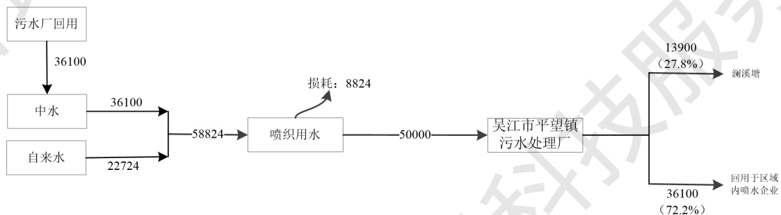
图2-3 技改前吴江市日通纺织有限公司水平衡图 t/a
