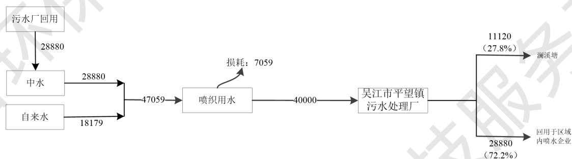
图2-7技改前吴江市丰帛纺织有限公司水平衡图 t/a
