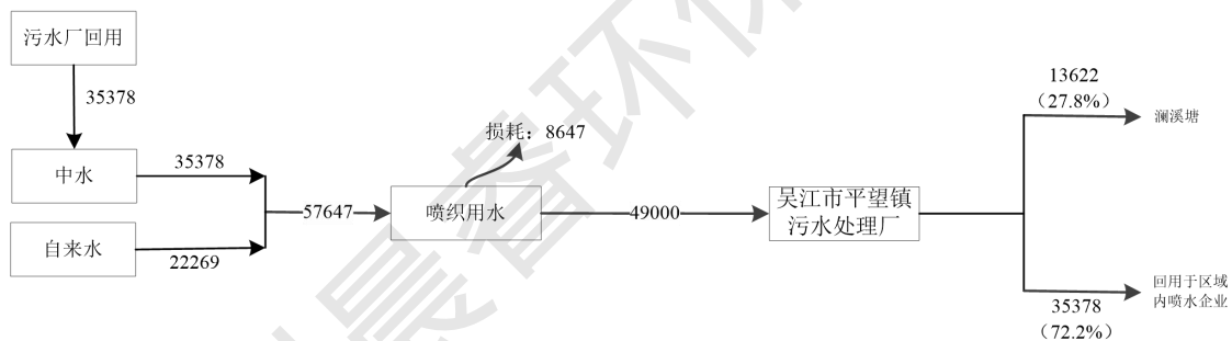
图2-4 技改前苏州久诚纺织有限公司水平衡图 t/a
