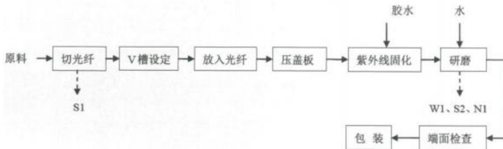
图2-3 现有项目工艺流程图
