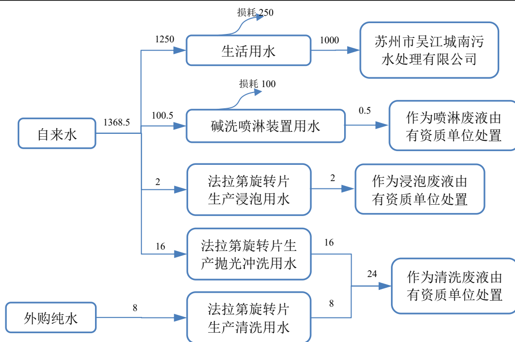
图 2-1 本项目用排水平衡图 (单位: t/a)
