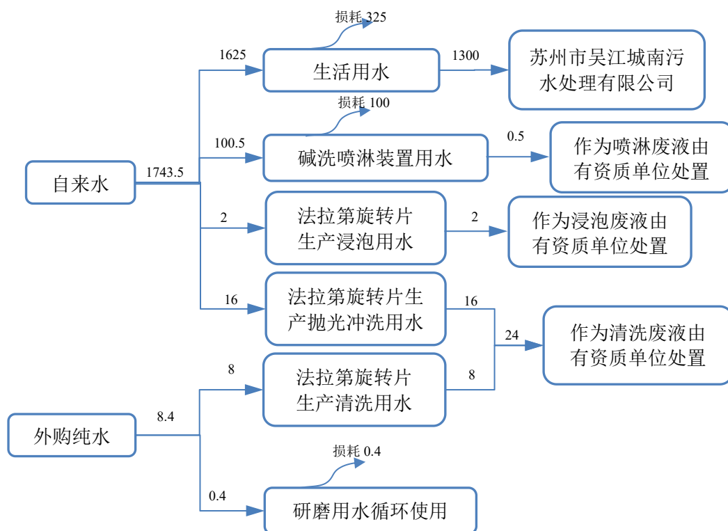
图 2-2 扩建后全厂用排水平衡图 (单位: t/a)
