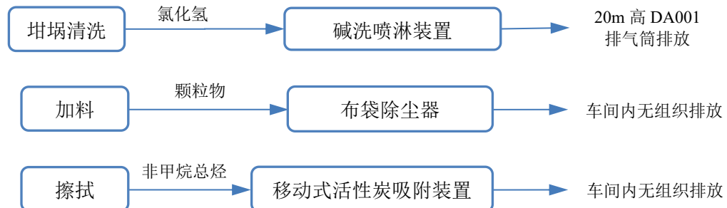
图 4-1 本项目废气收集及处理方式图
