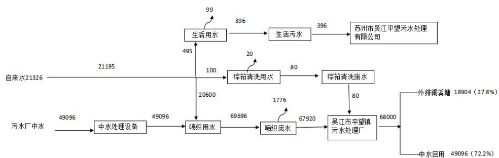
图2-3搬迁后苏州财生达纺织有限公司水平衡图 t/a
