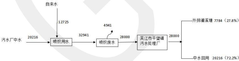
图2-2搬迁前苏州烨宇纺织有限公司水平衡图 t/a
