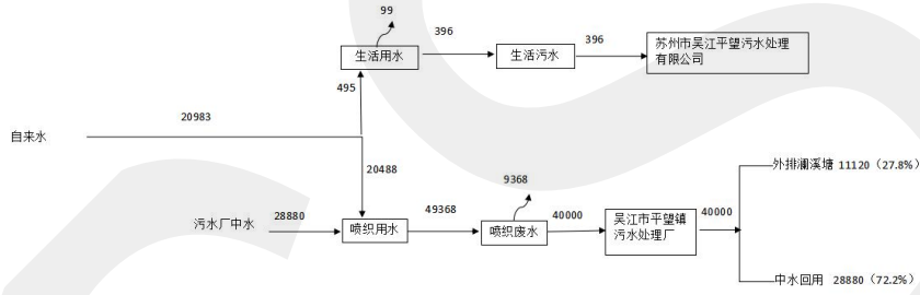
图2-1搬迁前苏州财生达纺喷头织有限公司水平衡图 t/a
