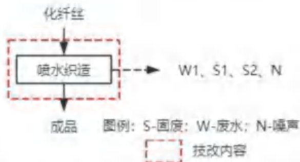
图 2-3 生产工艺流程及产污环节示意图
