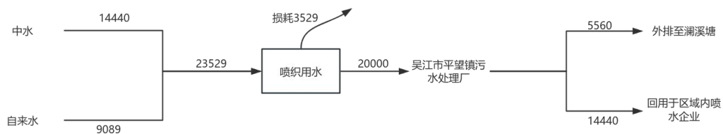
图2-4技改前吴江新吕喷织有限公司水平衡图 t/a
