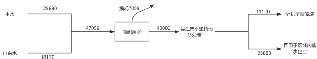
图2-6技改前吴江市集杰织造有限公司水平衡图 t/a
