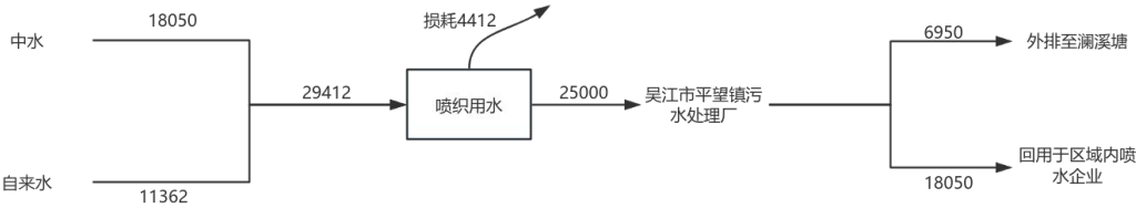
图2-2技改前吴江市银云布业有限公司水平衡图 t/a
