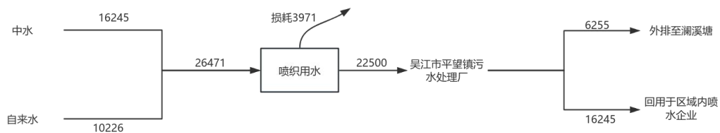
图2-5技改前苏州守宝纺织有限公司水平衡图 t/a
