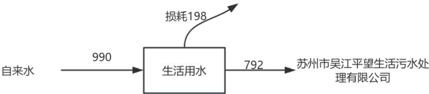
图2-1技改前吴江市立加喷织有限公司水平衡图 t/a
