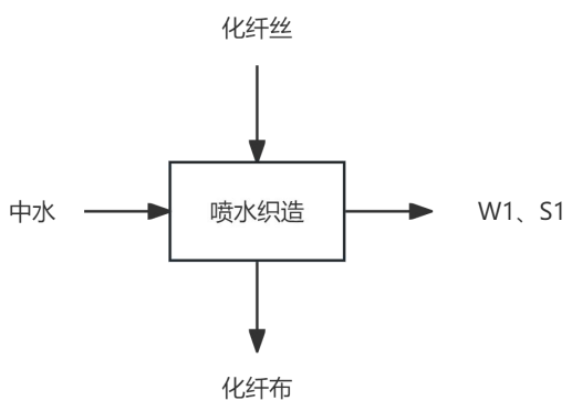
图 2-11 现有项目生产及产污环节示意图
