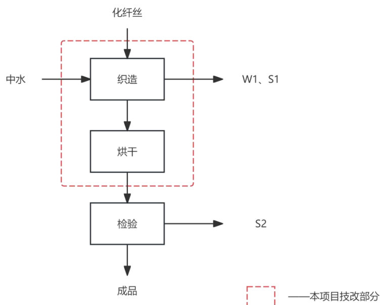
图 2-7 生产工艺流程及产污环节示意图
