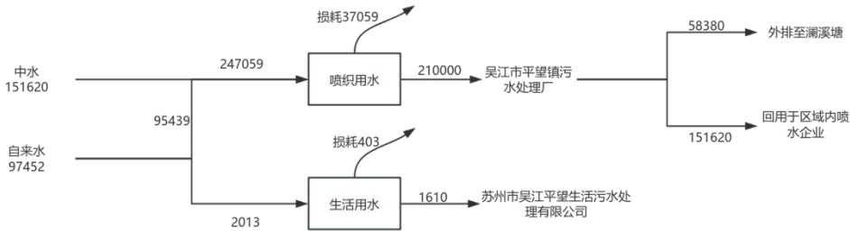
图2-1技改前吴江新明宇织造有限公司水平衡图 t/a
