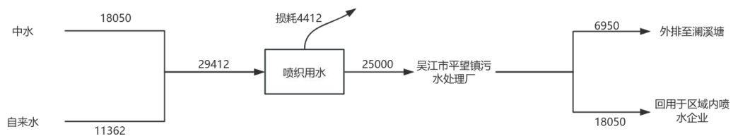
图2-2技改前苏州宇希纺织厂水平衡图 t/a
