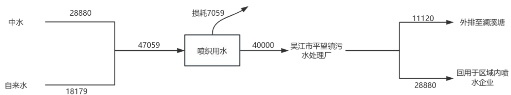
图2-3技改前苏州恒忠纺织有限公司水平衡图 t/a
