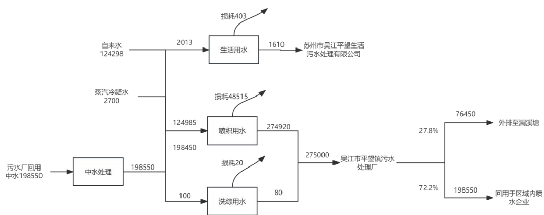
图2-6技改后水平衡图 t/a
