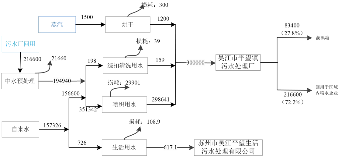
图2-2技改后水平衡图 t/a
