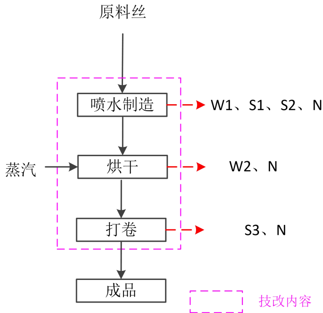
图 2-3 生产工艺流程及产污环节示意图
