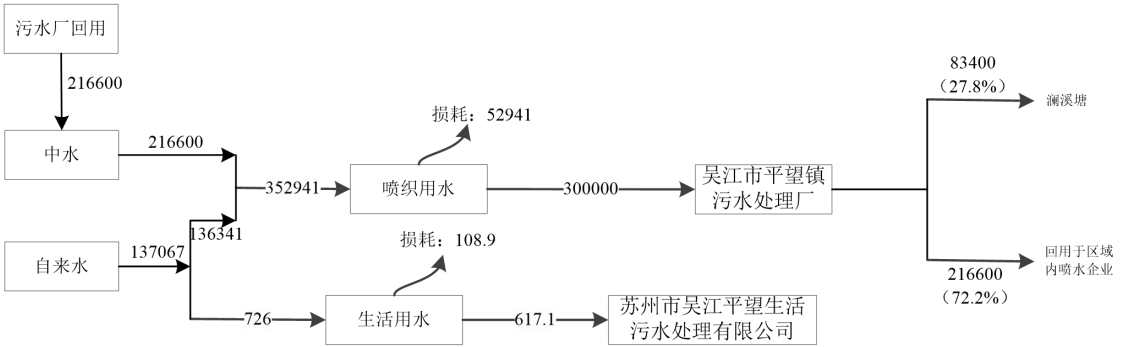
图2-1技改前吴江市春秋纺织品有限公司水平衡图 t/a
