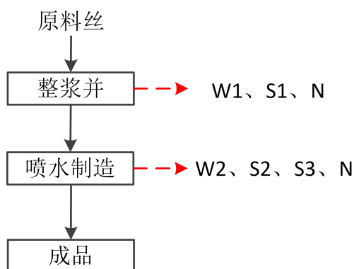
图 2-5 现有项目生产及产污环节示意图
