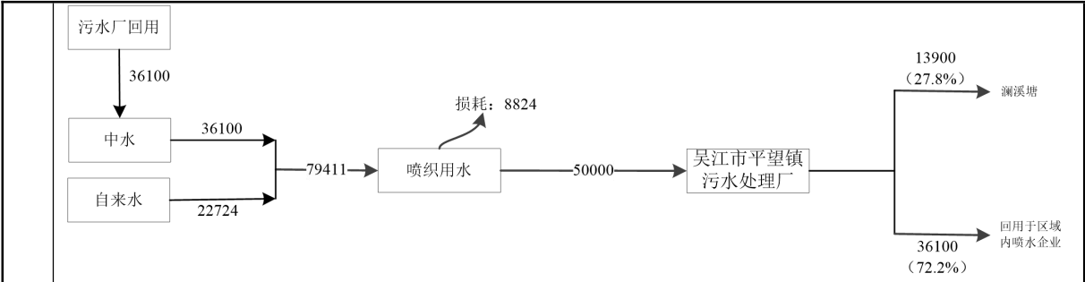
图2-9技改前苏州鹏凯织造有限公司水平衡图 t/a
