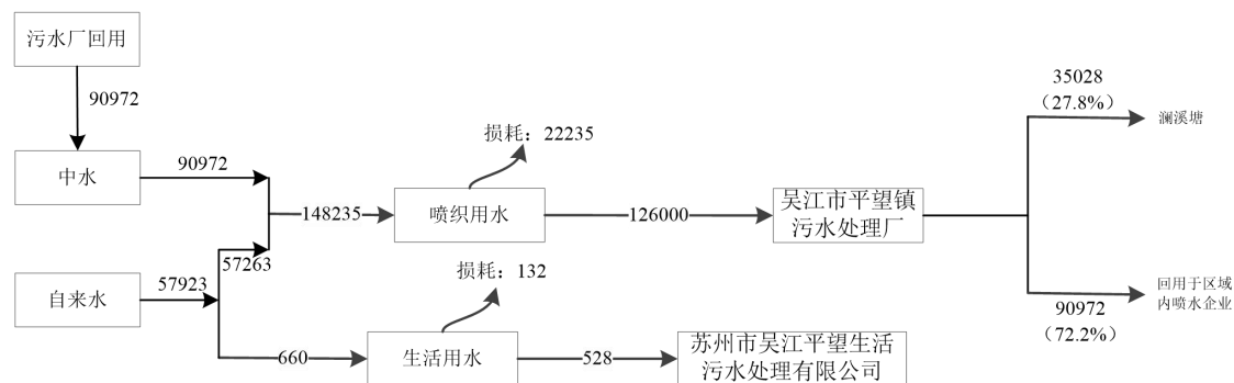
图2-1技改前吴江市凯越纺织有限公司水平衡图 t/a
