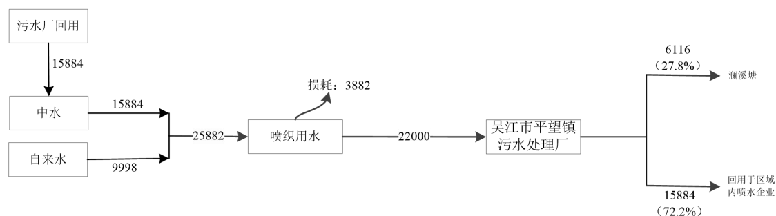
图2-3技改前苏州市奥纶纺织有限公司水平衡图 t/a
