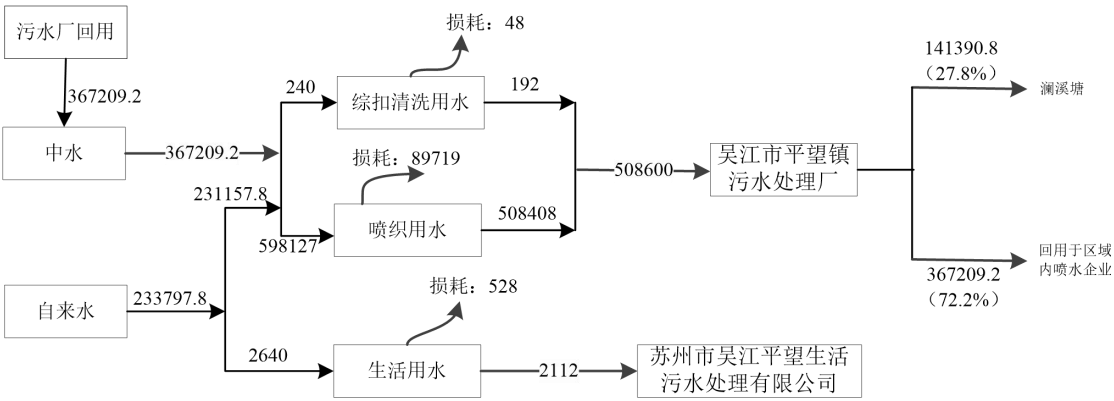
图2-9技改后水平衡图 t/a
