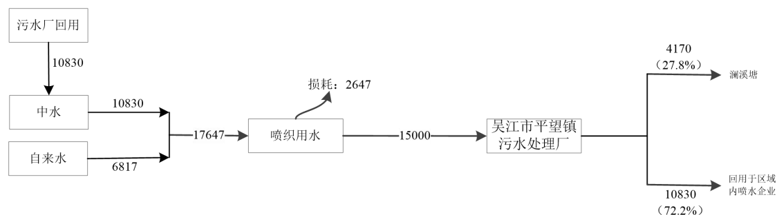
图2-4技改前苏州杰明圣纺织有限公司水平衡图 t/a
