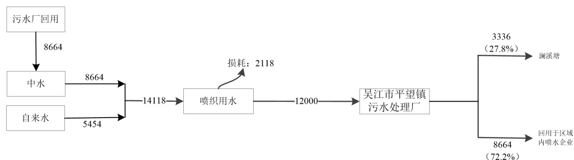
图2-2技改前苏州市奥拓纺织有限公司水平衡图 t/a
