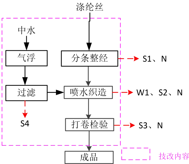
图 2-4 生产工艺流程及产污环节示意图
