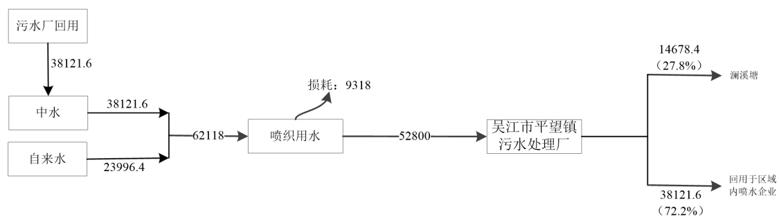
图2-3技改前吴江市月涵纺织厂水平衡图 t/a
