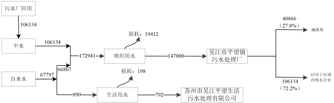
图2-1技改前苏州昇涛纺织科技有限公司水平衡图 t/a
