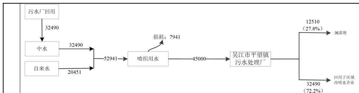
图2-2技改前苏州广申飞纺织有限公司水平衡图 t/a
