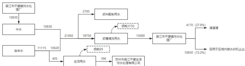
图2-6 技改前吴江翔丰丝绸整理有限公司水平衡图 (t/a)
