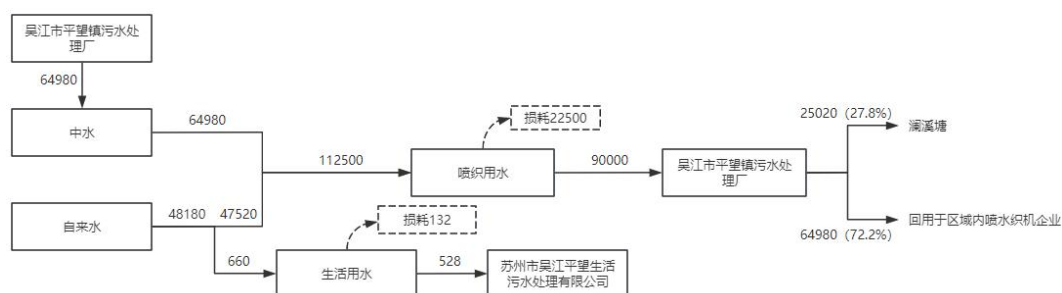
图2-1技改前苏州拓胜织造有限公司水平衡图 (t/a)
