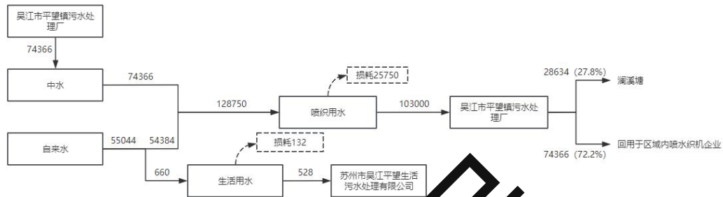
图2-3 技改前吴江市棧良纺织有限公司水平衡图 (t/a)
