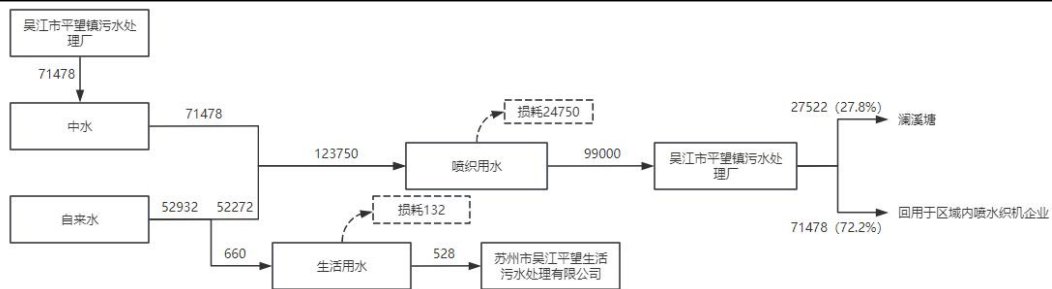
图2-2 技改前吴江市旭浩纺织有限公司水平衡图 (t/a)
