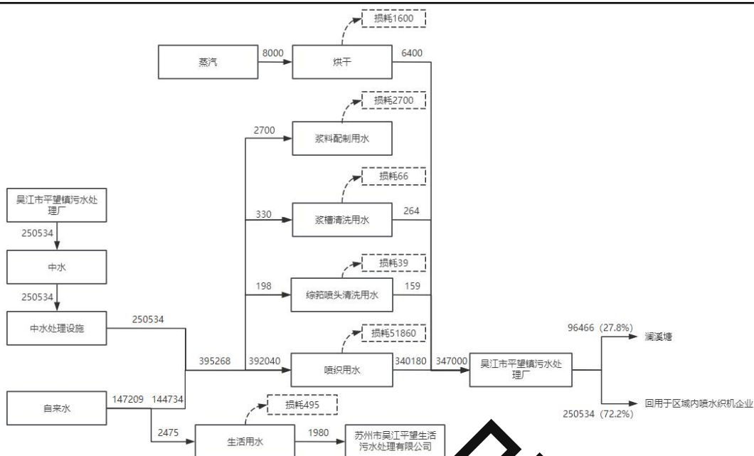
图 2-7 技改后全厂水平衡图 (t/a)
