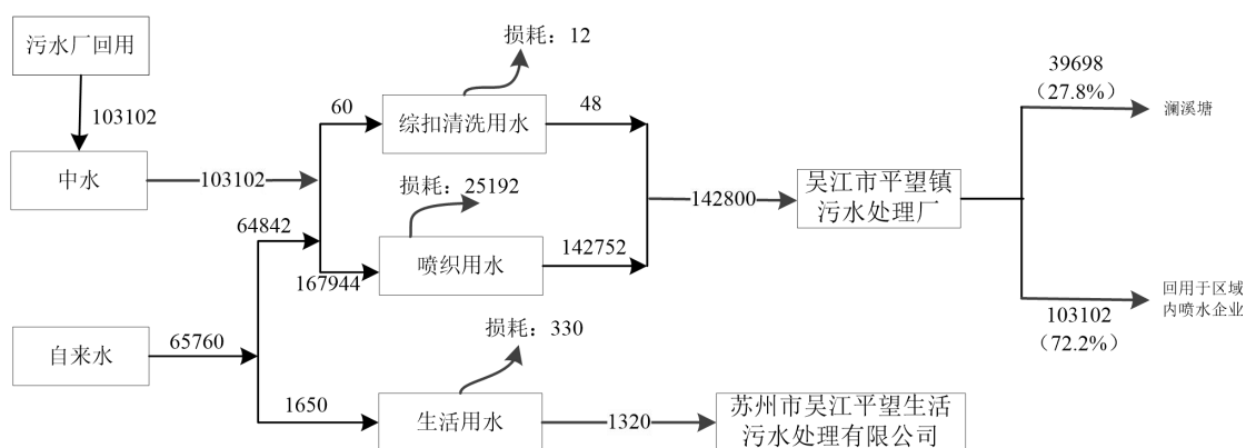
图2-3 搬迁后吴江市鼎灵纺织有限公司水平衡图 t/a
