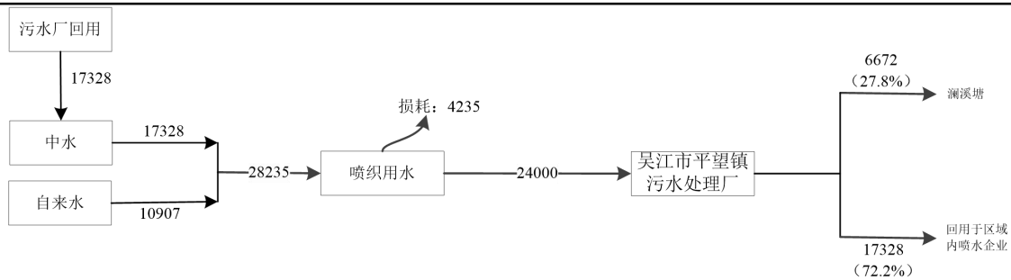
图2-2 搬迁前苏州永氏恒纺织有限公司水平衡图 t/a
