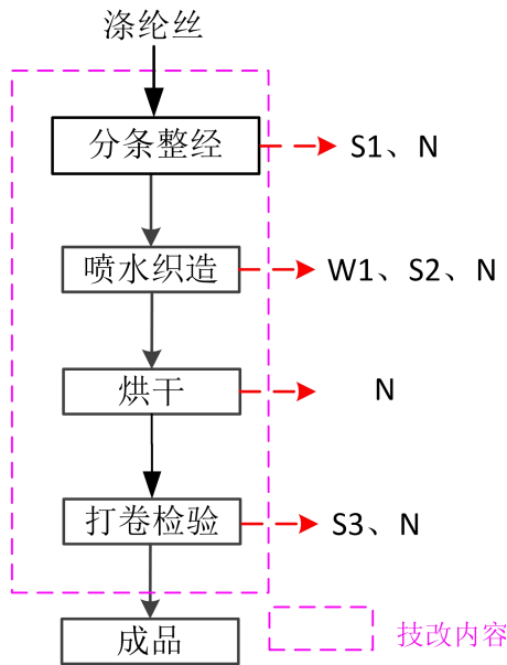
图 2-4 生产工艺流程及产污环节示意图
