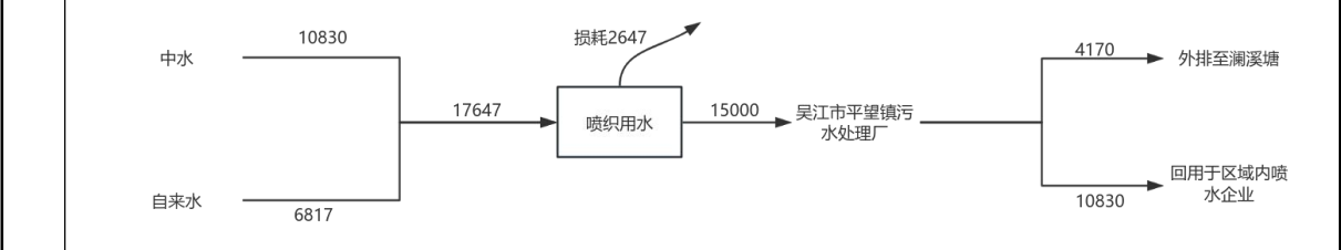
图2-3 技改前苏州新盼纺织有限公司水平衡图 t/a
