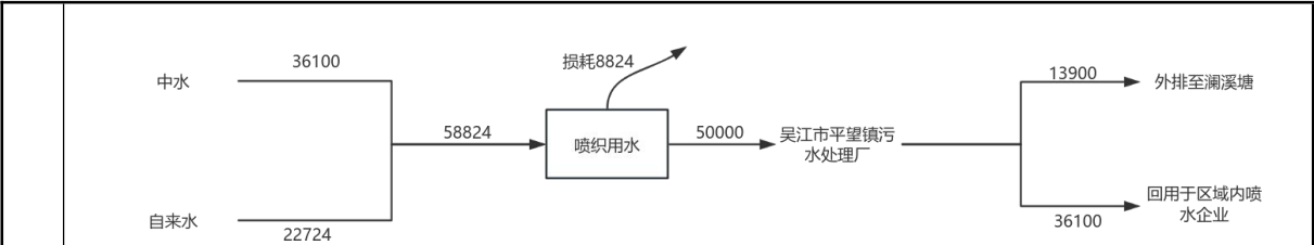
图2-2 技改前吴江市丽杏纺织有限公司水平衡图 t/a
