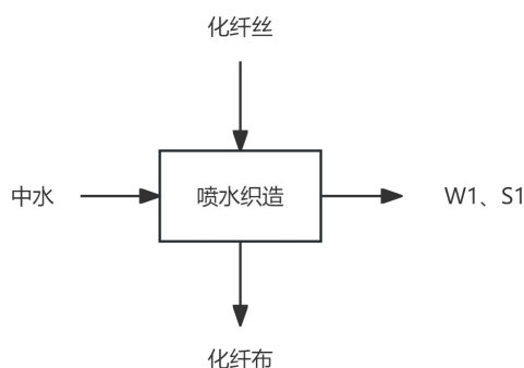
图 2-9 现有项目生产及产污环节示意图
