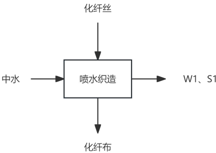
图 2-10 现有项目生产及产污环节示意图
