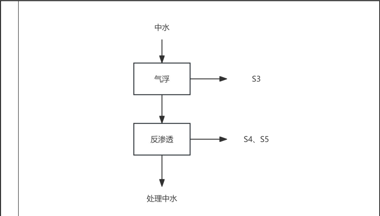
图 2-8 中水处理工艺流程及产污环节示意图
