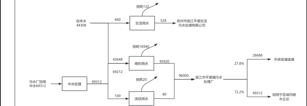
图2-6 技改后水平衡图 t/a
