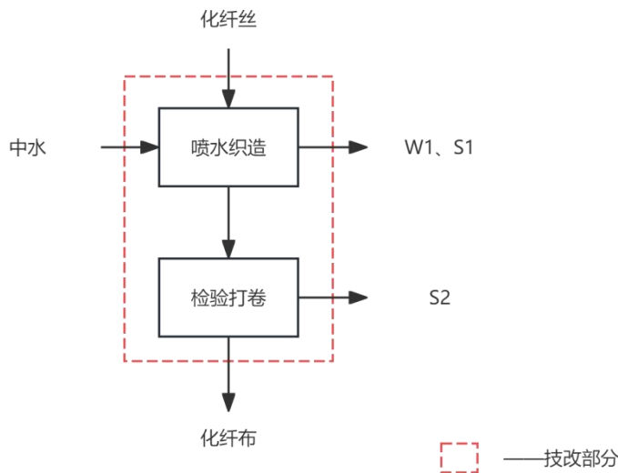
图 2-7 生产工艺流程及产污环节示意图
