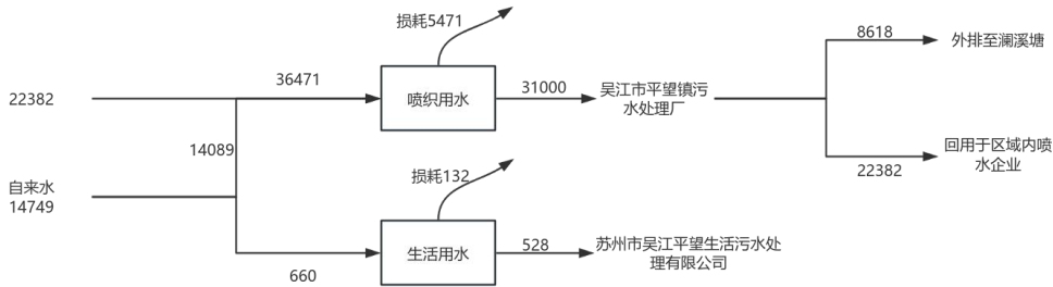
图2-1技改前吴江市向前纺织有限公司水平衡图 t/a
