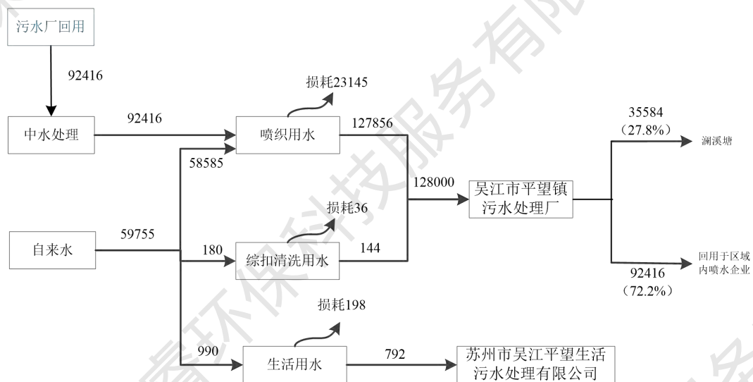
图2-3 技改后全厂水平衡图 t/a
