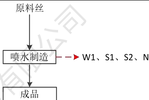
图 2-6 现有项目生产及产污环节示意图
