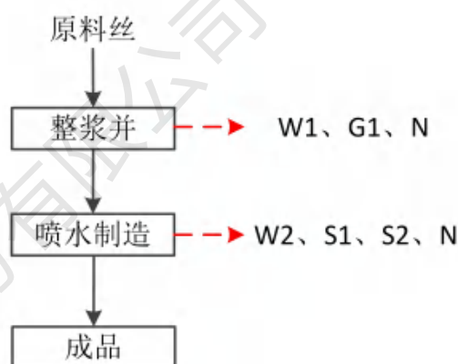
图 2-7 现有项目生产及产污环节示意图
