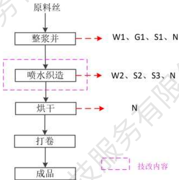
图 2-4 生产工艺流程及产污环节示意图
