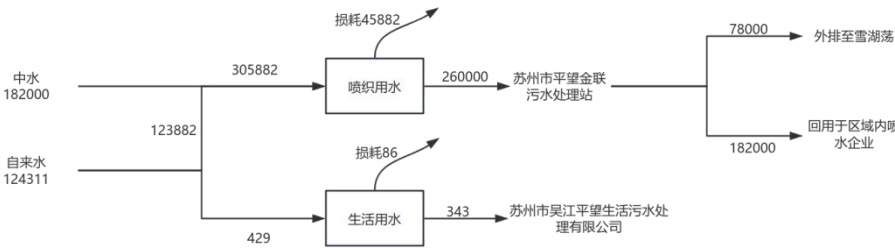
图2-1技改前吴江市晴华织造厂水平衡图 t/a
