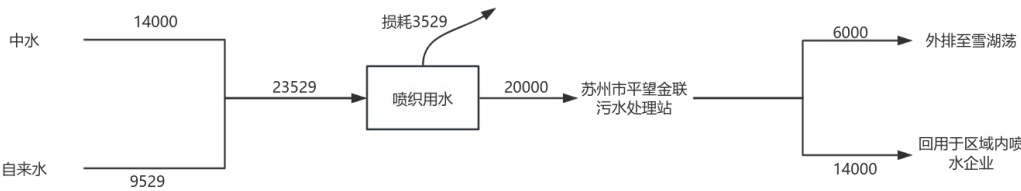
图2-3技改前苏州雄运纺织有限公司水平衡图 t/a
