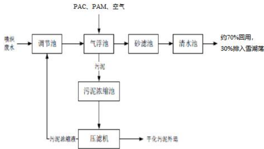
图 4-1 苏州市平望金联污水处理站处理工艺流程
