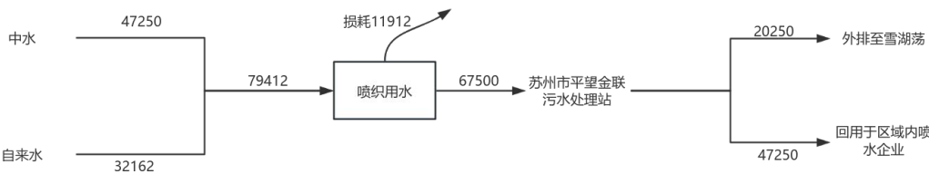
图2-2技改前吴江缘怡纺织有限公司水平衡图 t/a
