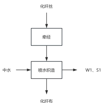
图 2-12 现有项目生产及产污环节示意图
