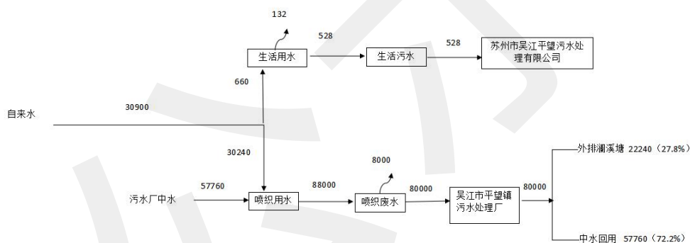
图2-1技改前吴江市益田纺织有限公司水平衡图 t/a
