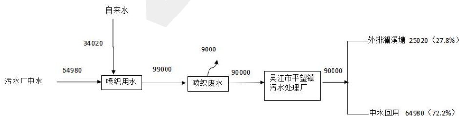
图2-1技改前吴江市益田纺织有限公司水平衡图 t/a
