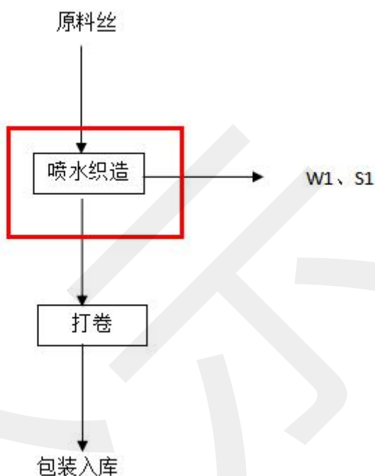
图 2-4 生产工艺流程及产污环节示意图
