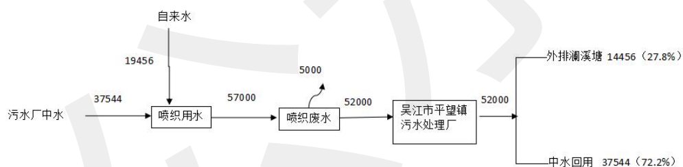
图2-3技改前吴江鑫创纺织有限公司水平衡图 t/a
