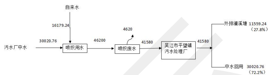
图2-2技改前吴江市锋澜纺织有限公司水平衡图 t/a
