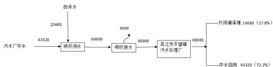
图2-1技改前苏州绣春纺织有限公司水平衡图 t/a
