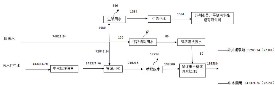
图2-5技改后吴江市超梦织造有限公司水平衡图 t/a
