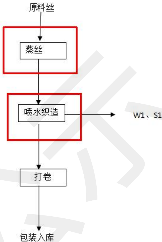
图 2-6 生产工艺流程及产污环节示意图
