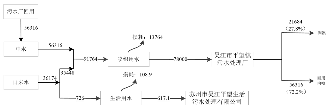
图2-1技改前吴江市友邦纺织品有限公司水平衡图 t/a
