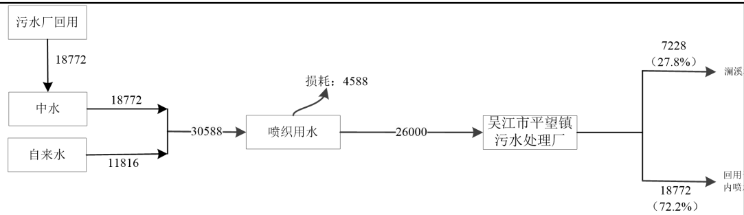
图2-6 技改前吴江市广永纺织有限公司水平衡图 t/a
