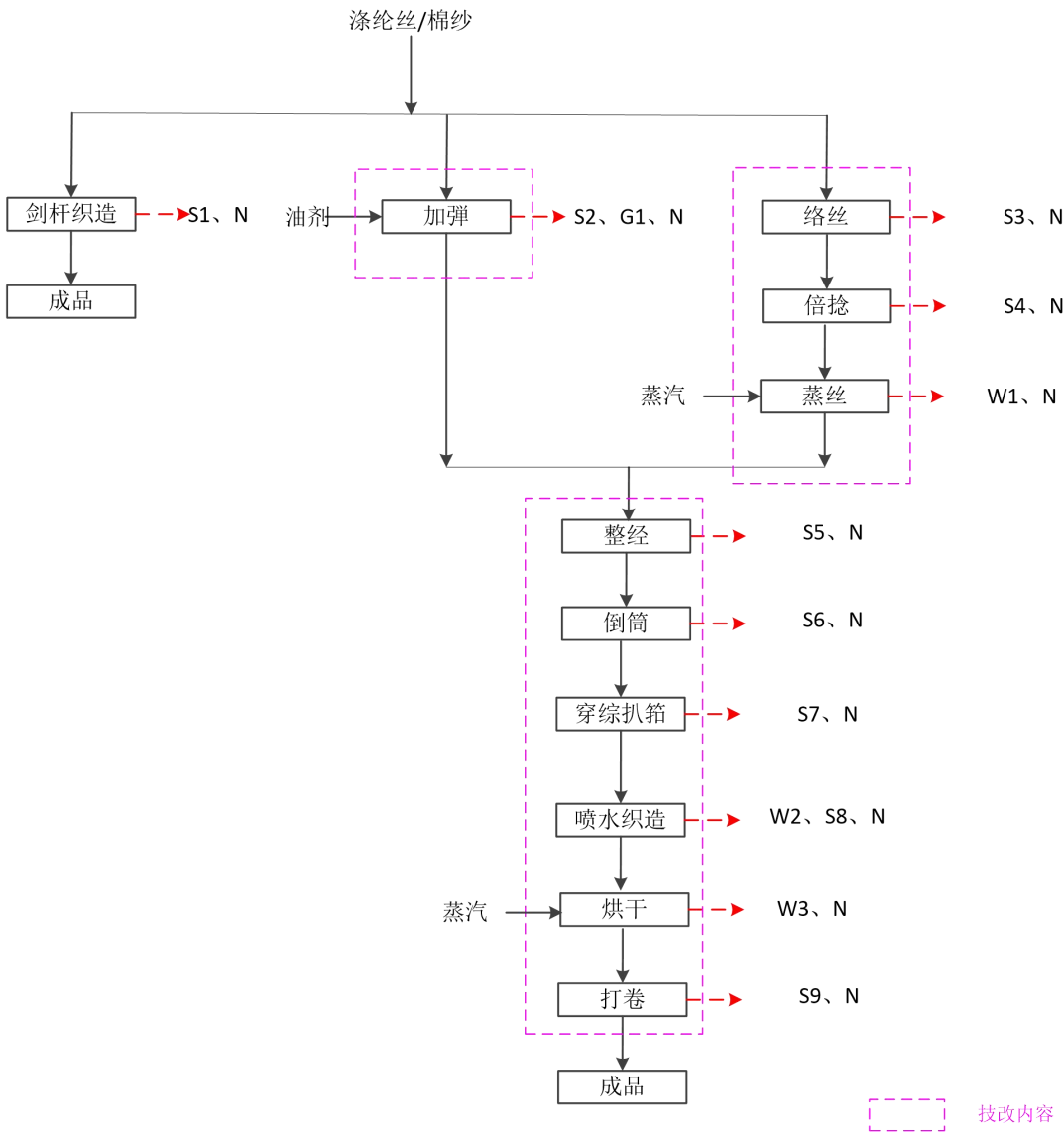
图 2-11 生产工艺流程及产污环节示意图 G-废气 S-固废 W-废水 -本次改建部分
