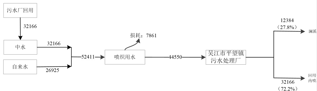
图2-3 技改前苏州市高柏纺织有限公司水平衡图 t/a
