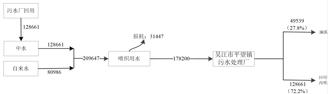
图2-9 技改前吴江市超瑞纺织有限公司水平衡图 t/a
