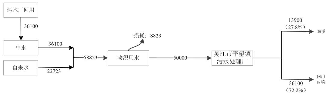
图2-7 技改前吴江市万兴利纺织厂水平衡图 t/a
