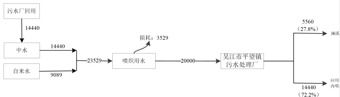
图2-5 技改前苏州市嘉拓纺织有限公司水平衡图 t/a
