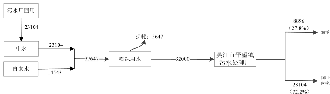
图2-4 技改前苏州市中川纺织有限公司水平衡图 t/a
