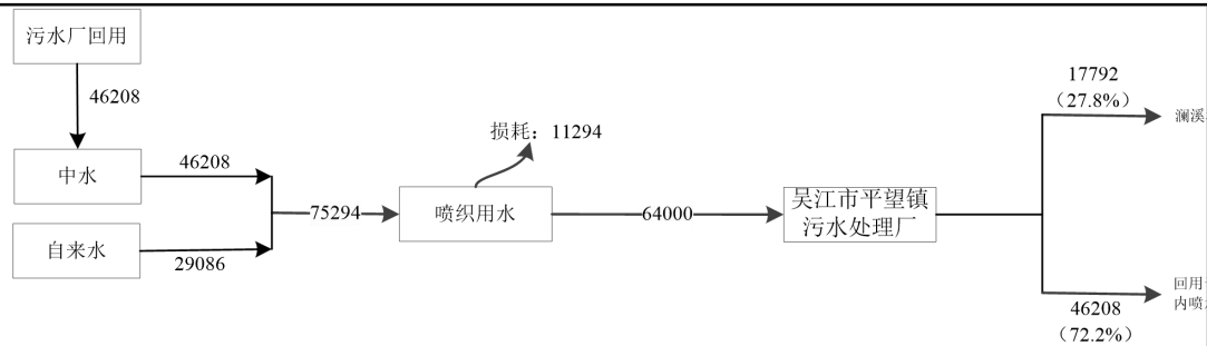
图2-2 技改前苏州市利尔达纺织有限公司水平衡图 t/a
