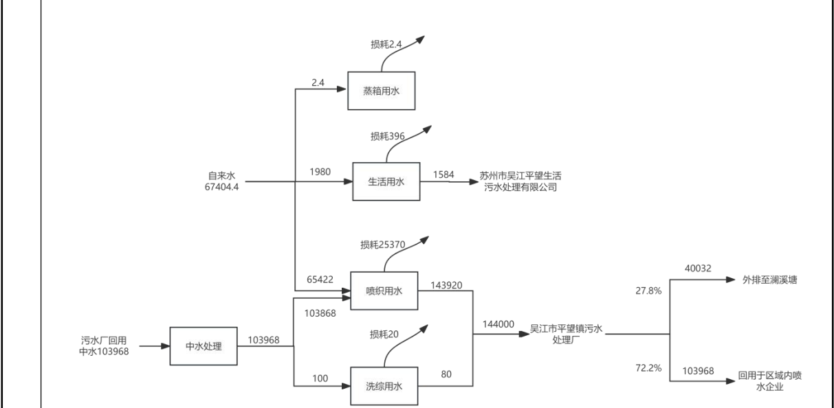
图2-4技改后水平衡图 t/a
