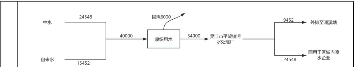
图2-2技改前吴江伟松塑胶有限公司水平衡图 t/a
