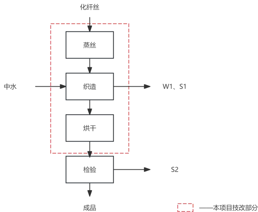
图 2-4 生产工艺流程及产污环节示意图
