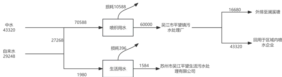
图2-1技改前吴江天星纺织有限公司水平衡图 t/a
