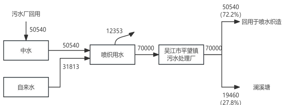
图2-1技改前吴江市贝腾纺织实业有限公司水平衡图 t/a
