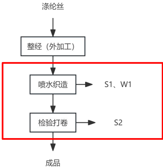
图 2-4 生产工艺流程及产污环节示意图
