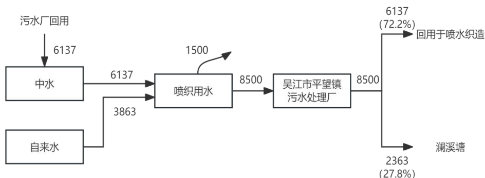
图2-2技改前苏州市坤华纺织有限公司水平衡图 t/a
