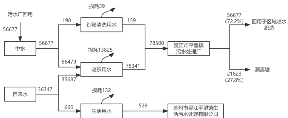
图2-3技改后水平衡图 t/a
