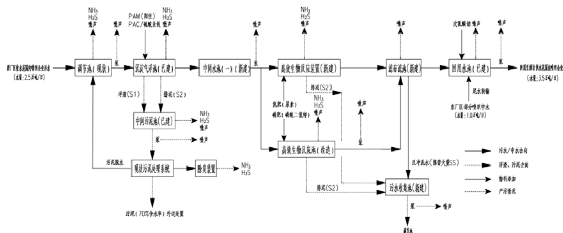
图 4-1 吴江市平望镇污水处理厂处理工艺流程
