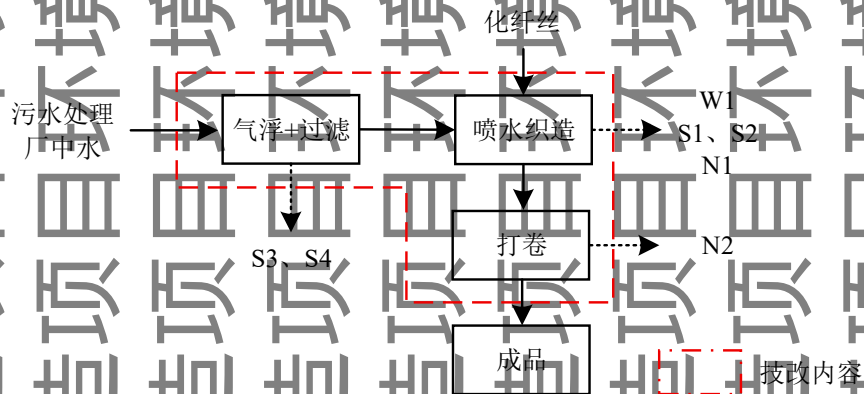
图 2-3 生产工艺流程及产污环节示意图
