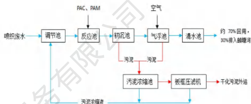
图 4-1 苏州市平望龙南污水处理站处理工艺流程
