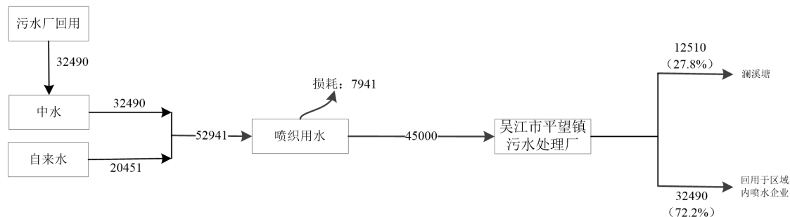
图2-2技改前吴江市胜旺纺织有限公司水平衡图 t/a
