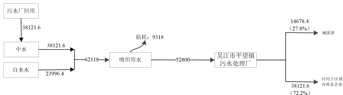
图2-3技改前吴江钱程纺织有限公司水平衡图 t/a
