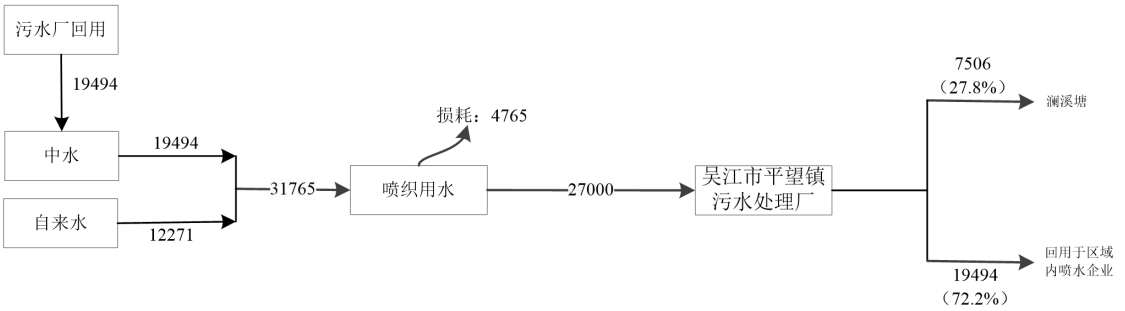
图2-2技改前苏州市佳祺纺织品有限公司水平衡图 t/a
