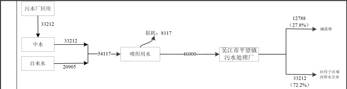
图2-7技改前苏州鑫昇纺织有限公司水平衡图 t/a
