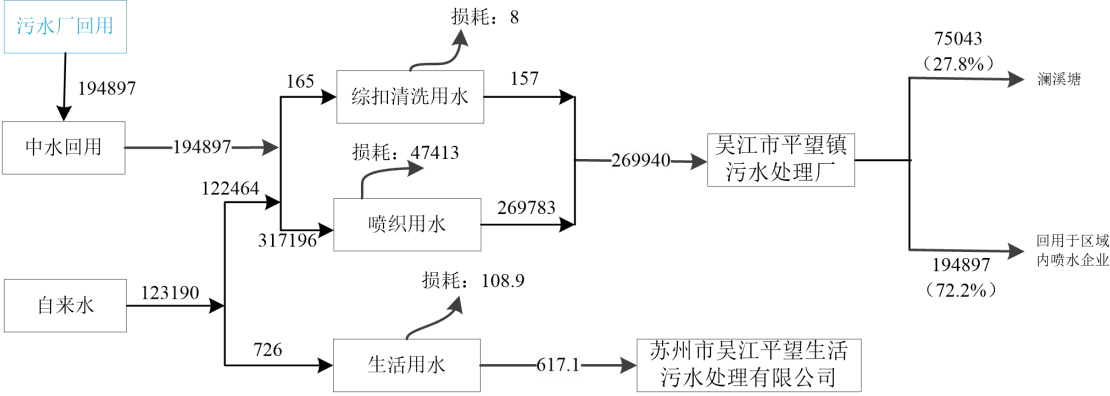
图2-8技改后水平衡图 t/a
