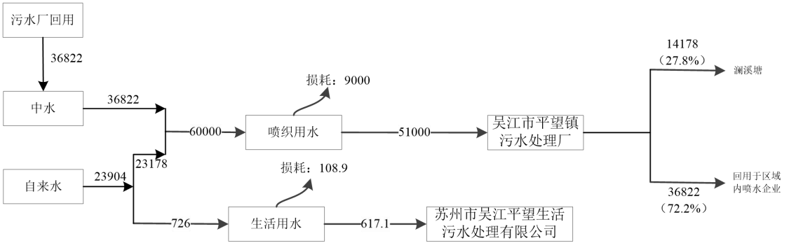
图2-1技改前吴江市中谊纺织有限公司水平衡图 t/a
