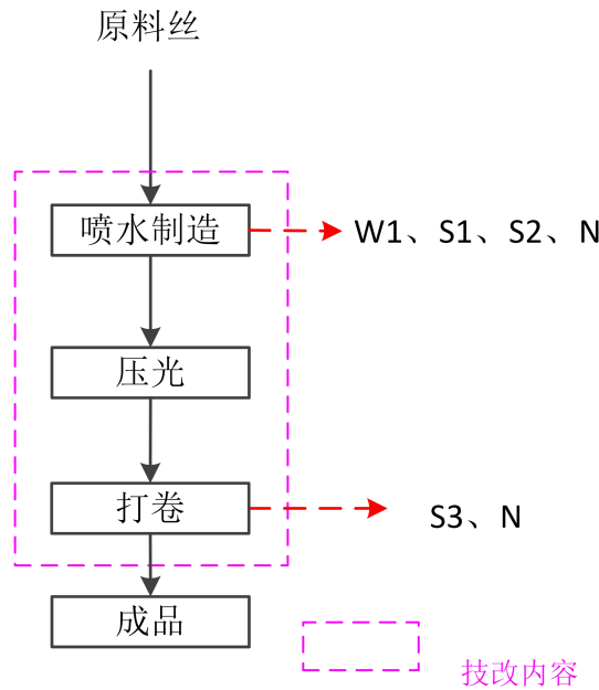
图 2-9 生产工艺流程及产污环节示意图
