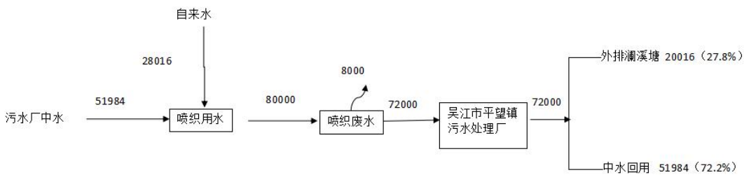
图2-3技改前吴江市昊昌喷织厂水平衡图 t/a
