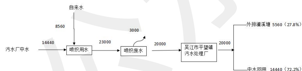
图2-6技改前苏州兴初纺织有限公司水平衡图 t/a
