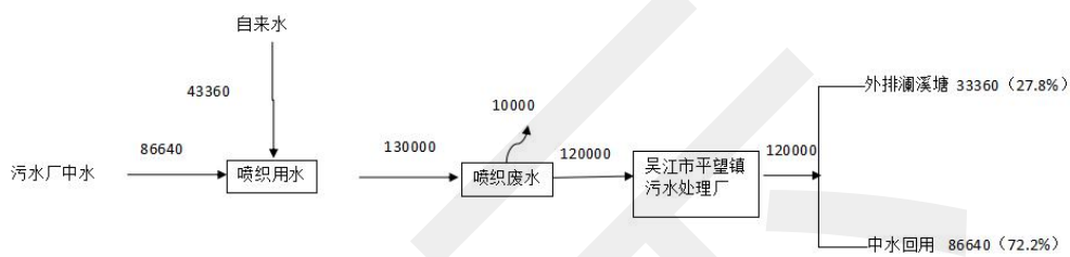
图2-1技改前吴江市创联纺织有限公司水平衡图 t/a
