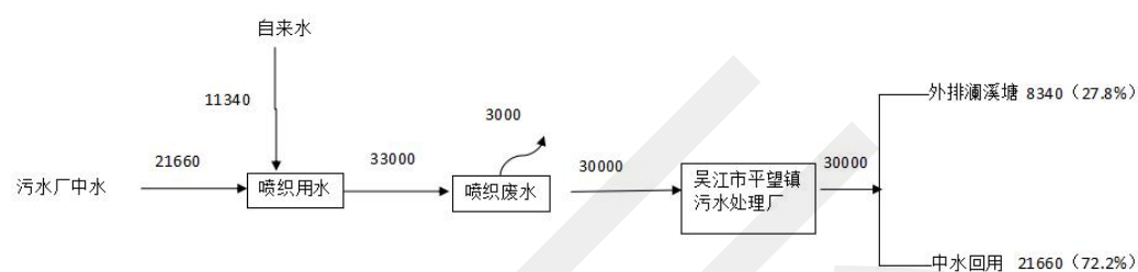
图2-5技改前吴江市三凤纺织厂水平衡图 t/a
