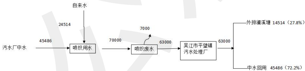
图2-2技改前吴江市富亿喷织有限公司水平衡图 t/a
