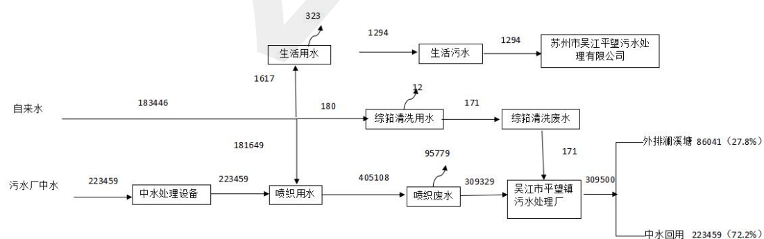
图2-6技改前苏州兴初纺织有限公司水平衡图 t/a
