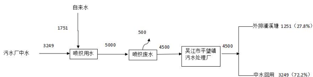
图2-4技改前吴江市瑞丰织造有限公司水平衡图 t/a
