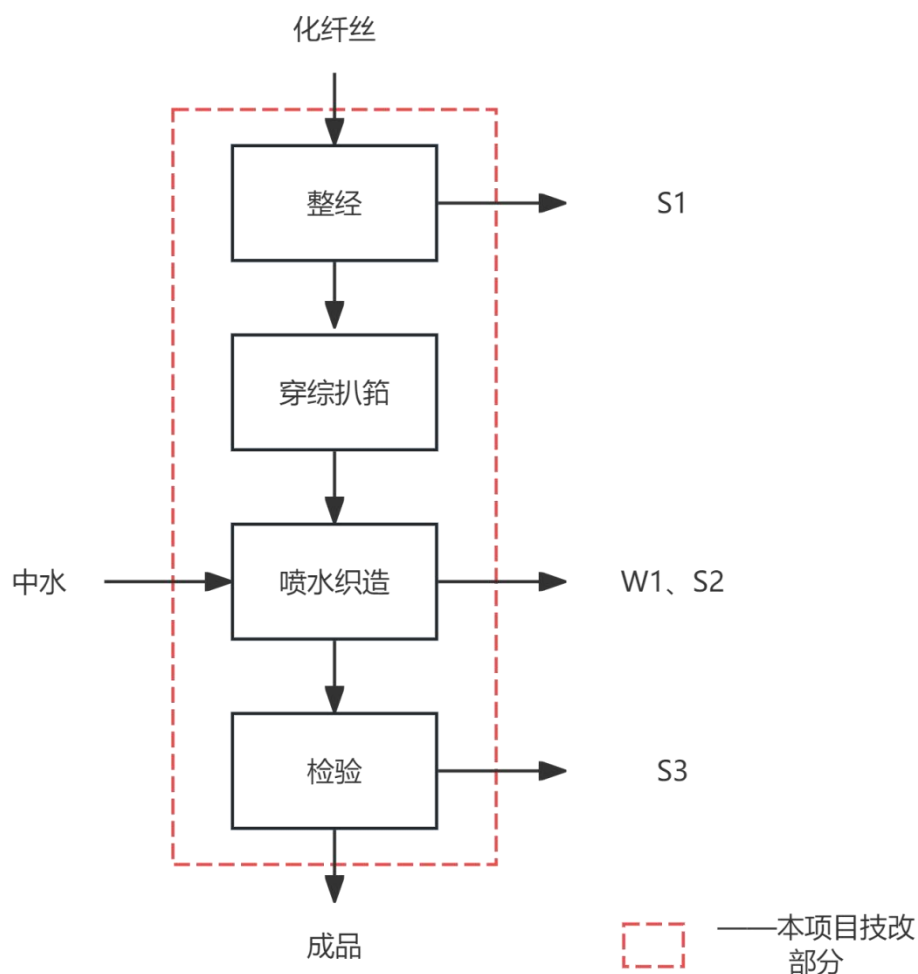
图 2-3 生产工艺流程及产污环节示意图
