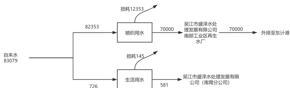
图2-1技改前荣博水平衡图 t/a
