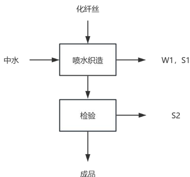
图 2-3 现有项目生产及产污环节示意图 W-废水 S-固废
