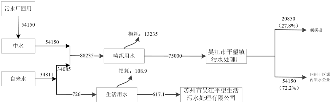
图2-1技改前吴江市平望镇天天磨毛复合厂水平衡图 t/a
