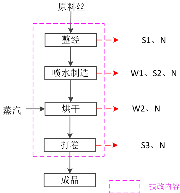
图 2-3 生产工艺流程及产污环节示意图
