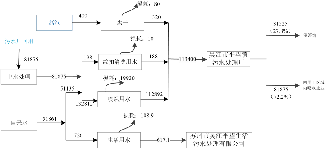
图2-3技改后水平衡图 t/a
