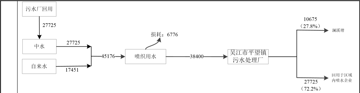
图2-2技改前吴江市宇毅纺织有限公司水平衡图 t/a
