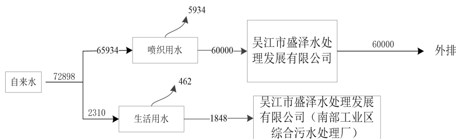
图2-1 改建前水平衡图 t/a
