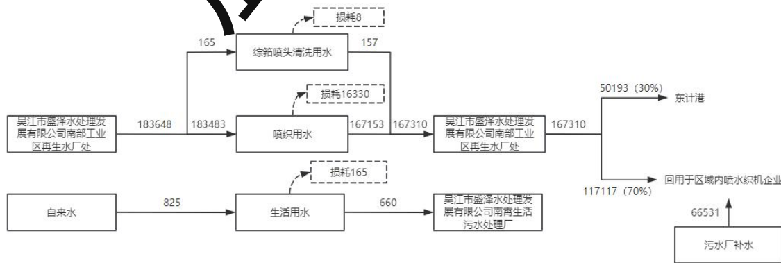
图2-1 技改后水平衡图t/a
