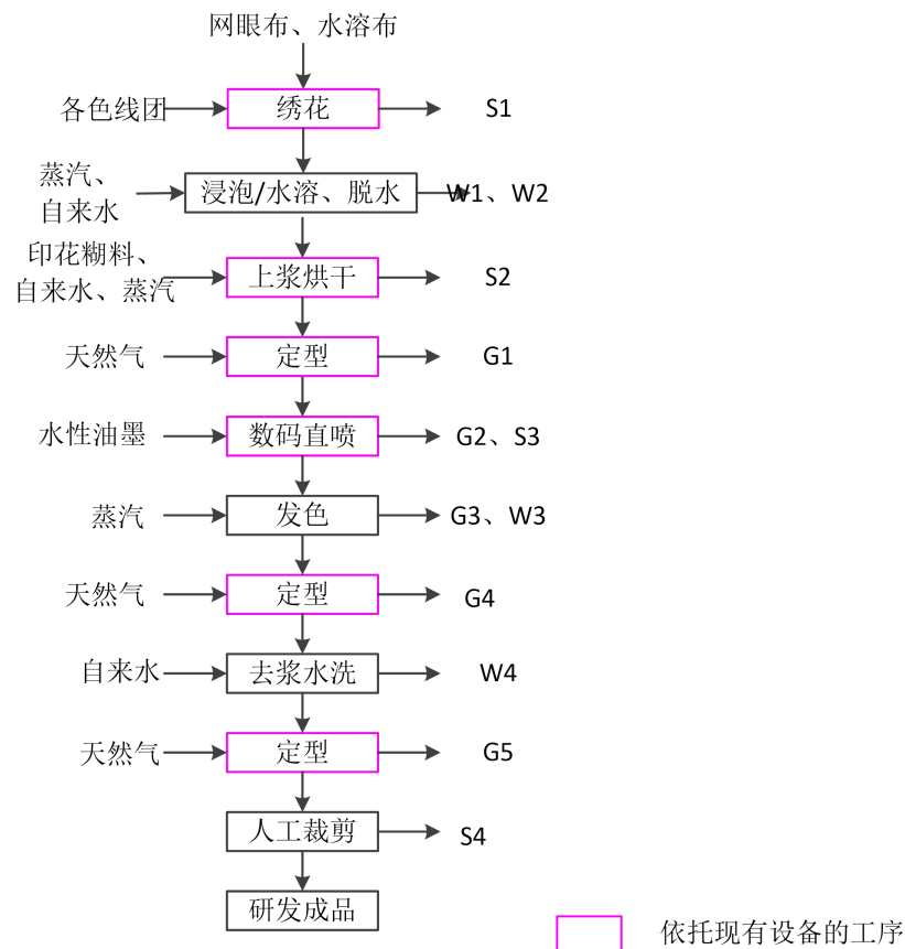
图2-2 工艺流程及产污环节示意图
