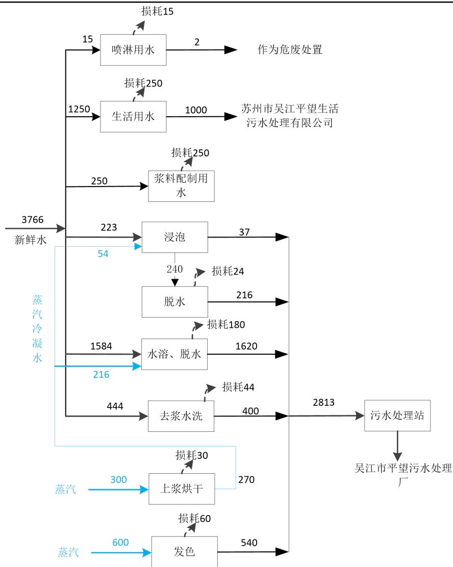
图 2-1 全厂水平衡 t/a
