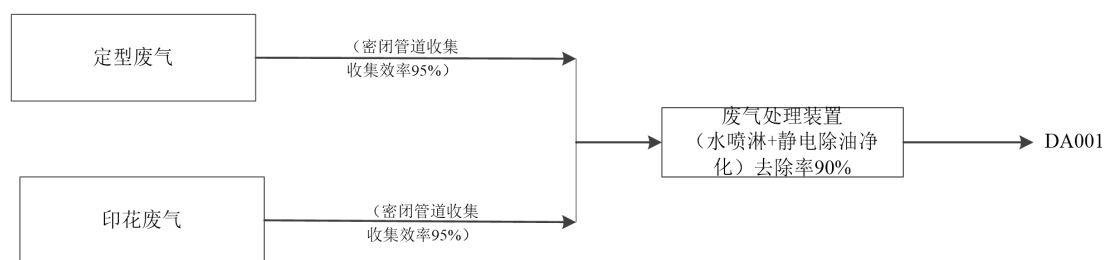
图 4-1 废气收集处理示意图
