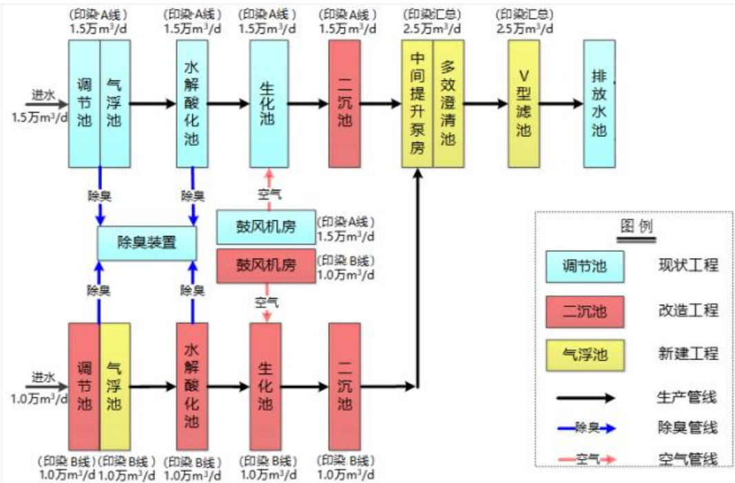
图 4-3 吴江市平望镇污水处理厂废水处理工艺流程图
