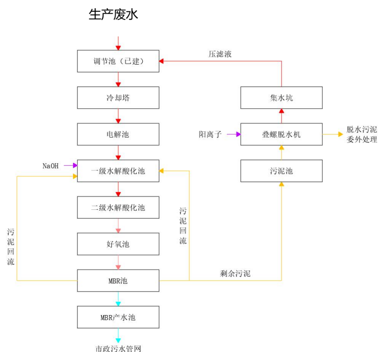
图 4-2 废水处理系统处理流程图
