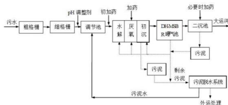
图 4-4 苏州市吴江平望生活污水处理有限公司废水处理工艺流程图
