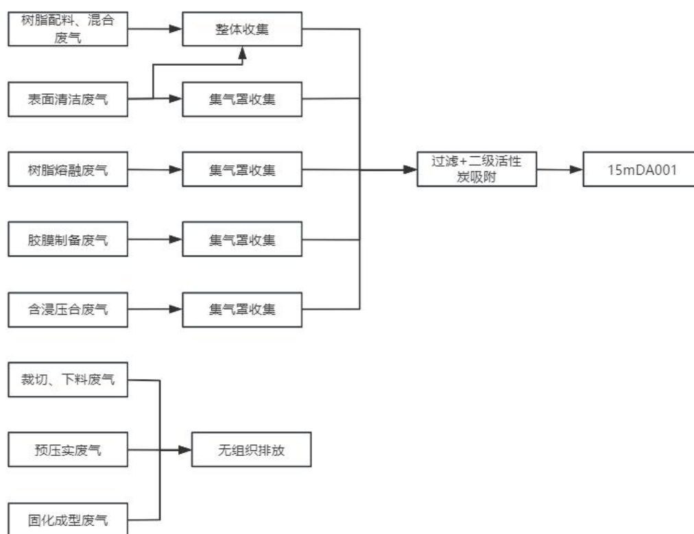
图 4-1 废气收集工艺流程图
