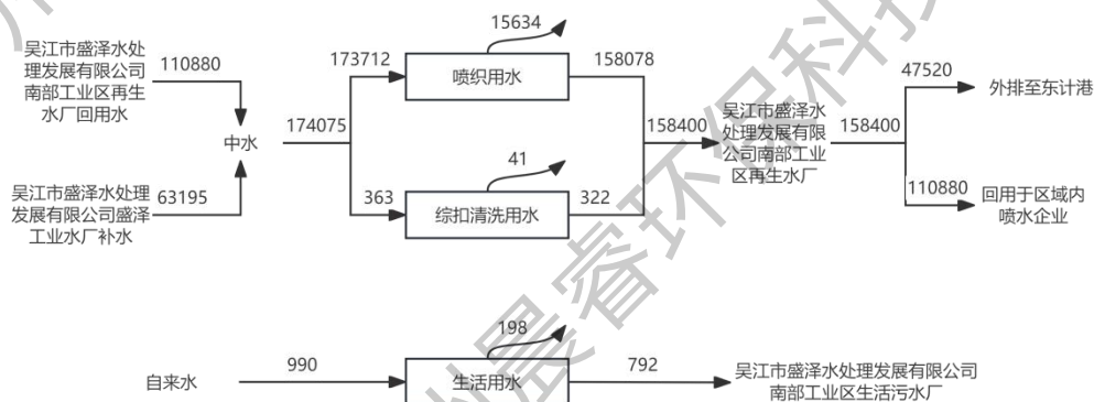
图2-2 改建后水平衡图 t/a
