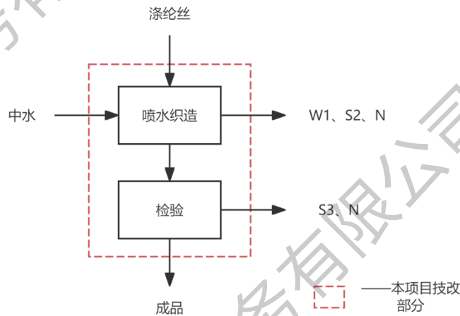
图 2-3 生产工艺流程及产污环节示意图
