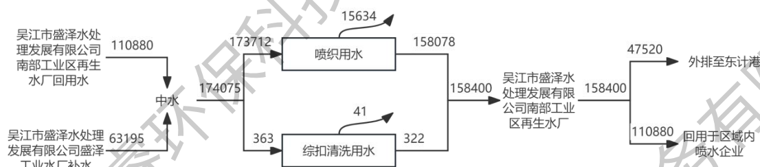
图2-1本项目水平衡图 t/a
