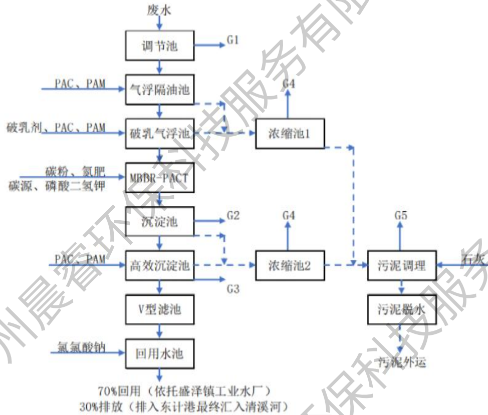
图 4-1 吴江市盛泽水处理发展有限公司南部工业区再生水厂处理工艺流程
